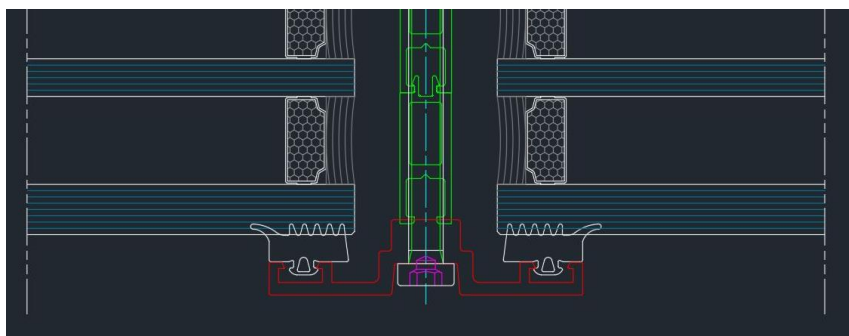
Slika 50. Omega profil
