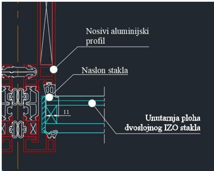
Slika 38. Naslon stakla na brtvu
