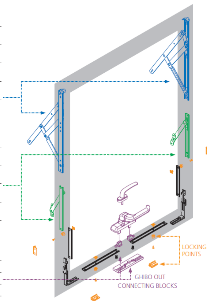
Slika 69. Shema sustava okova za otvaranje prema van proizvođača Giesse
