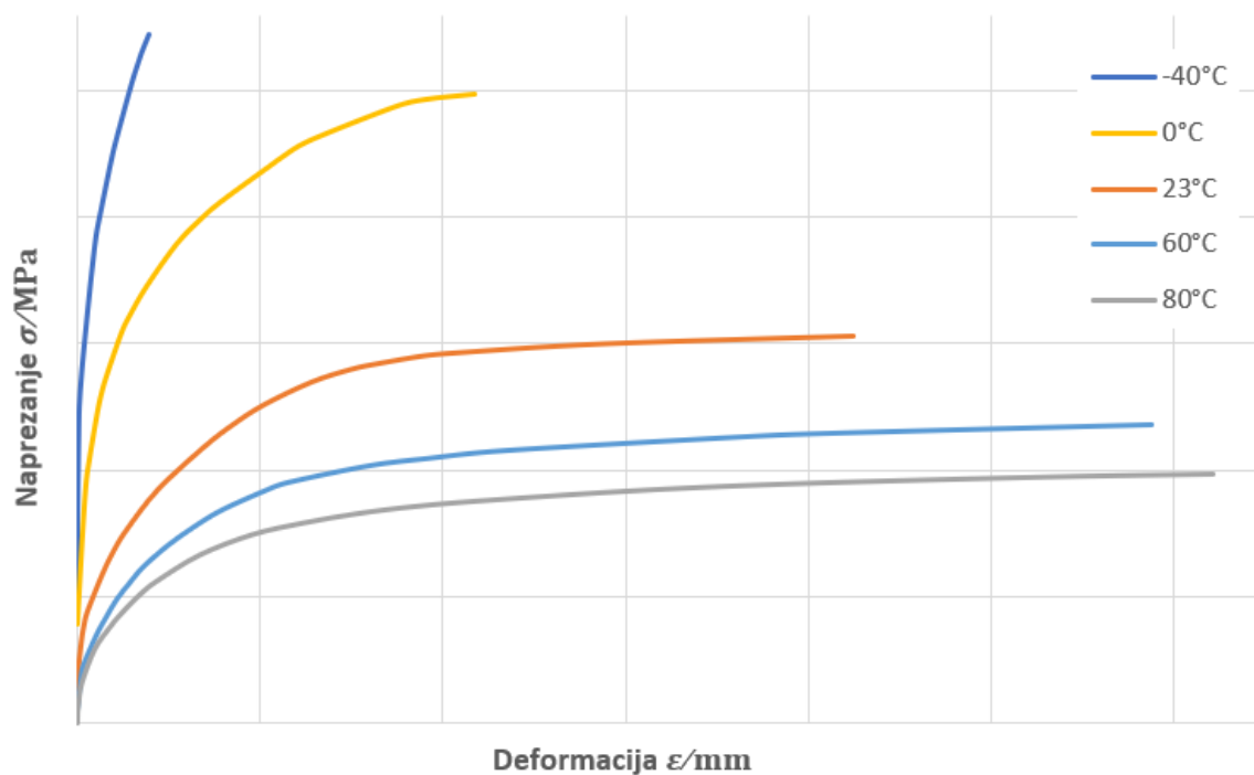
Slika 2.2. Simbolički graf naprežanje-deformacija materijala PAGF-13
