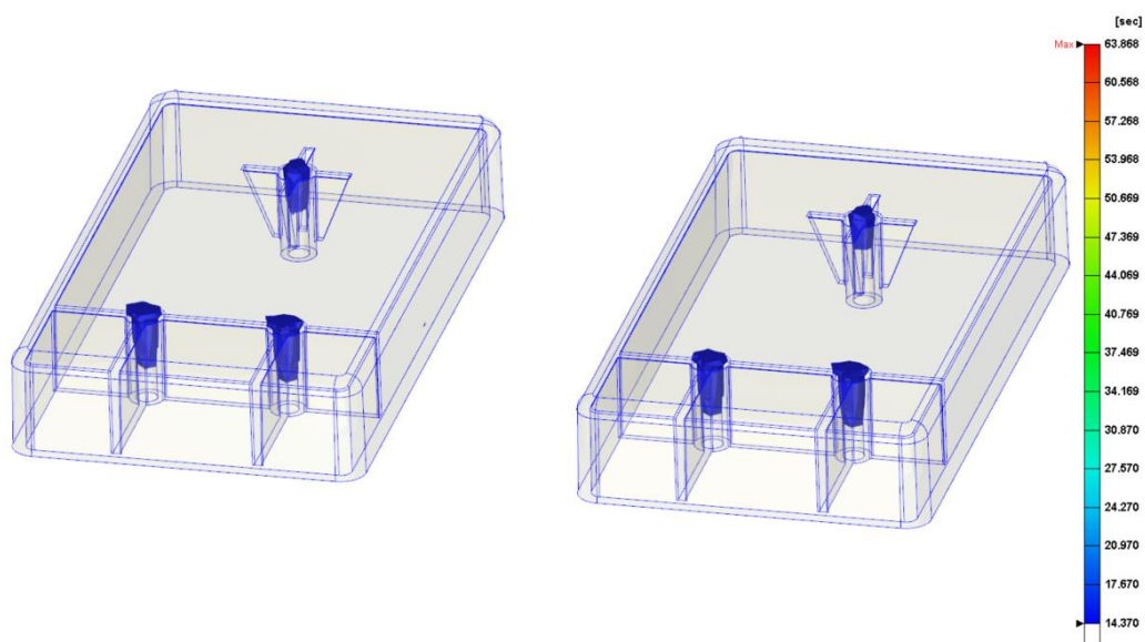
Slika 67. Procjena potrebnog vremena hlađenja otpreska uz primjenu konformalnog hlađenja
