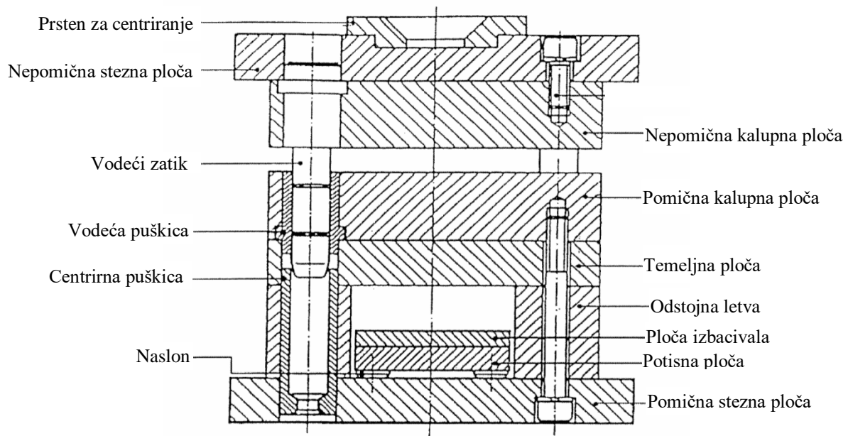
Slika 7. Kućište kalupa [5]
