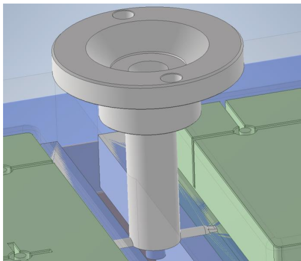
Slika 76. CAD model uljevnog sustava
