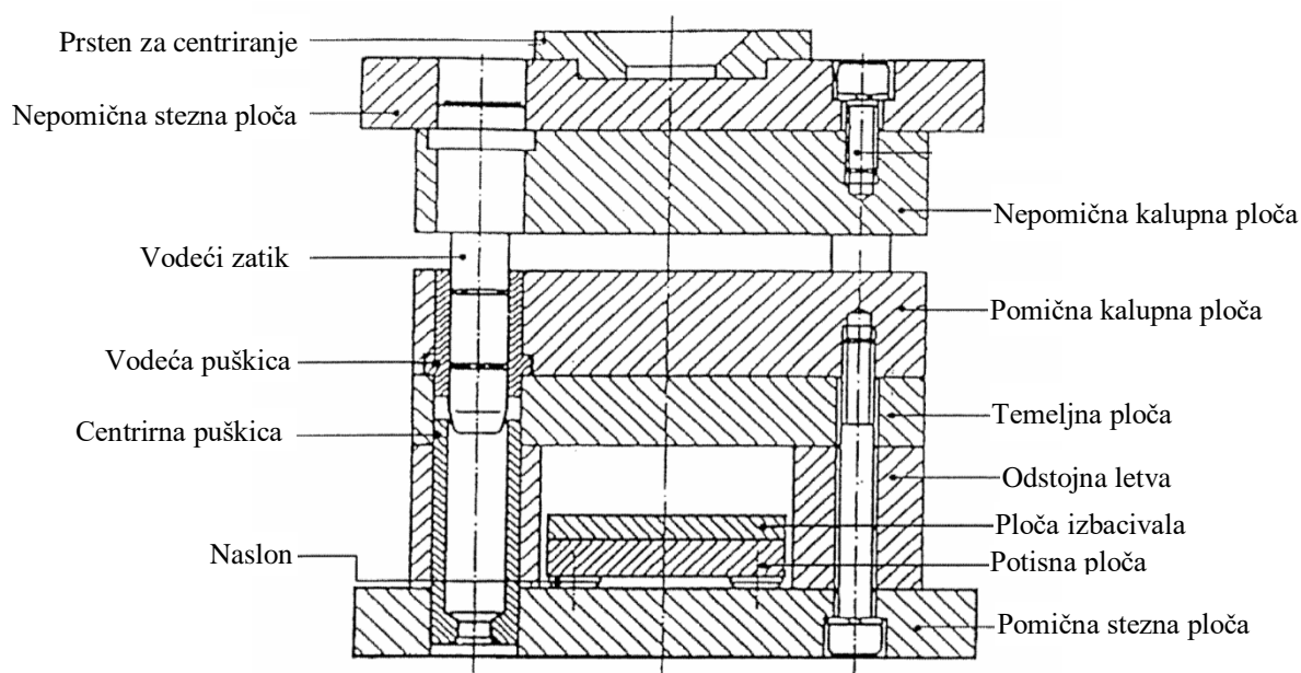
Slika 7. Kućište kalupa [5]
