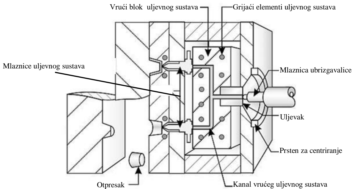
Slika 14. Vrući uljevni sustav [7]
