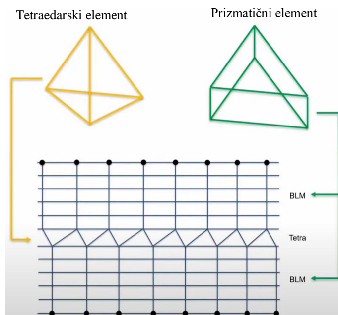
Slika 32. BLM mreža [18]
