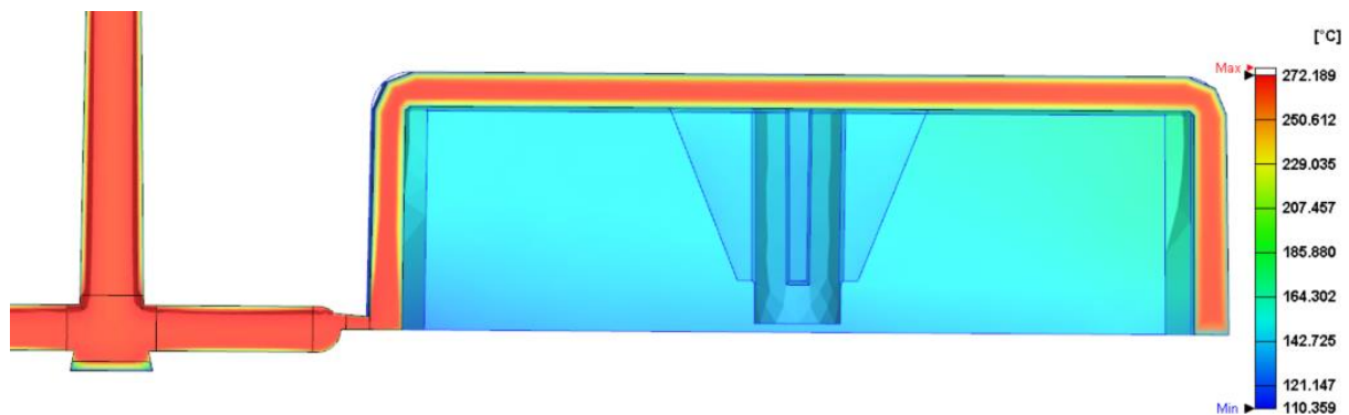
Slika 54. Raspored temperature taljevine po presjeku na kraju faze punjenja
