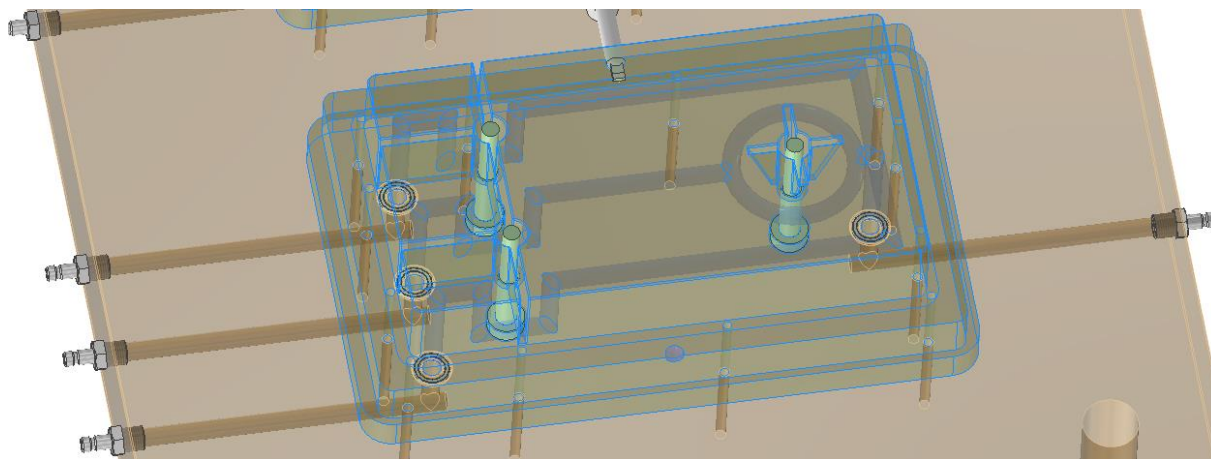
Slika 77. Donji krug za temperiranje kalupa
