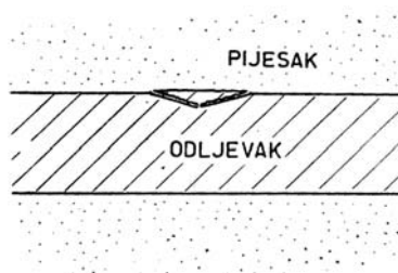
Slika 4.37 Presjek tipične odlupine [29]
