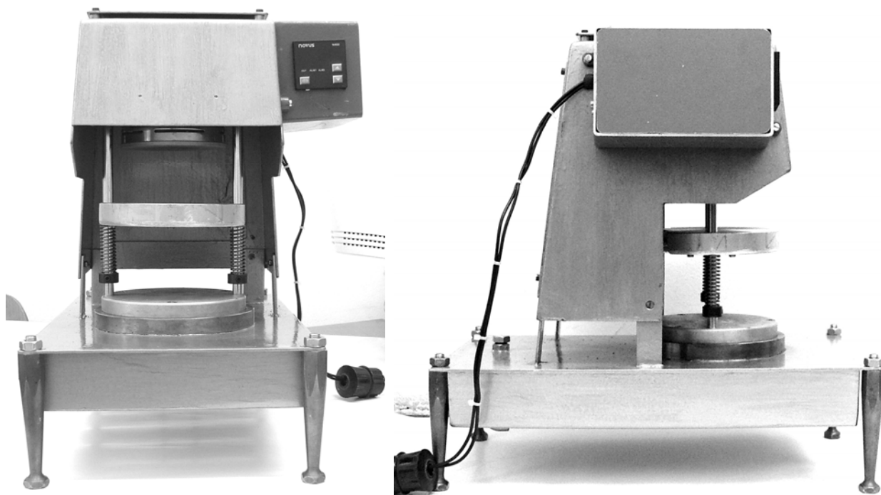
Slika 6.2 Fotografije mjernog uređaja za određivanje koeficijenta toplinske vodljivosti.
