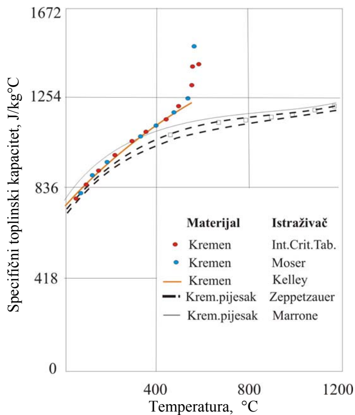
Slika 4.45 Specifični toplinski kapacitet kristala kremenja i kremenog pijeska [31]
