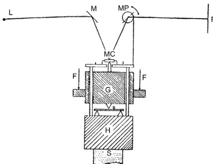
Slika 4.10 Uređaj za registraciju krivulje deformacija: FF-opterećenje, H-klip, B-kalibrirana poluga, S-uzorak, E-držač ogledala, MC-ogledalo, MR-rotaciono ogledalo, P-foto ploča, L-izvor svjetla, G-držač. [12]
