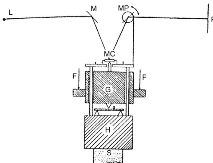
Slika 4.10 Uređaj za registraciju krivulje deformacija: FF-opterećenje, H-klip, B-kalibrirana poluga, S-uzorak, E-držak ogledala, MC-ogledalo, MR-rotaciono ogledalo, P-foto ploča, L-izvor svjetla, G-držać. [12]
