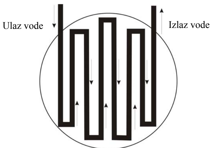
Slika 6.3 Shematski prikaz protjecanja vode kroz rashladni spremnik
