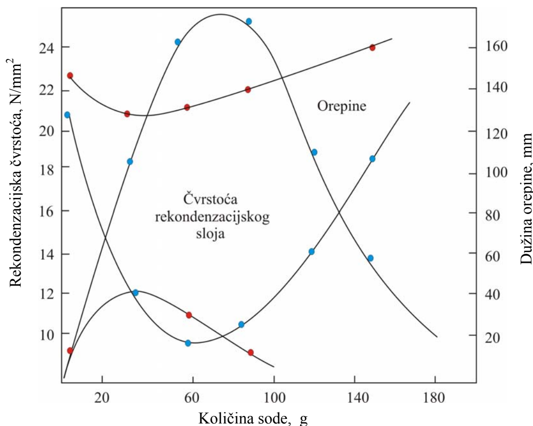
Slika 4.28 Odnos između rekondenzacijske čvrstoće, količine sode za aktivaciju i učestalosti pojave orepina za njemački (Gb) i indijski (Ib) bentonit [21].
