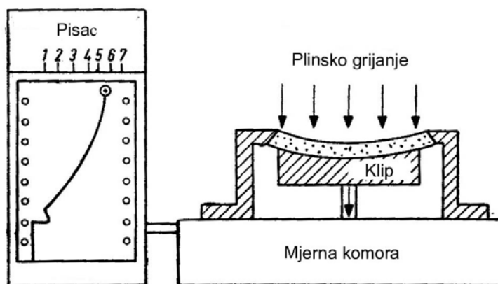
Slika 4.29 Shema uređaja za ispitivanje tlačnih napreznja [22]
