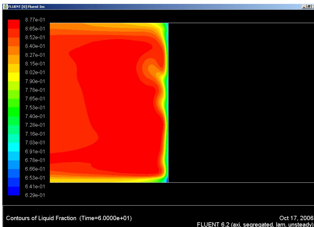
Slika 10.15 Skrućivanje nakon 60 s uz \lambda = 0,83 W/m K
