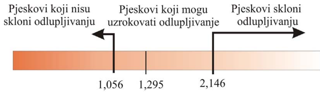
Slika 9.8 Shematski prikaz klasifikacija ljevačkih pjeskova s obzirom na sklonost odlupljivanju
