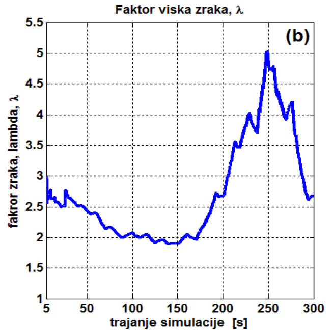
(b) Faktori viška zraka, lambda ( \lambda )
