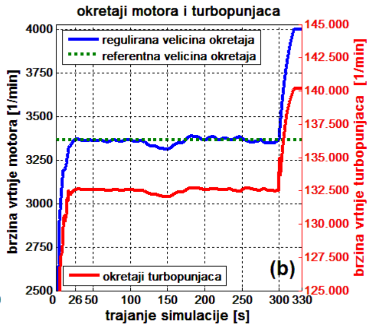
Slika 5.58 (b) Brzine vrtnje motora i turbopunjača
