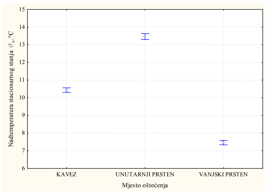
Slika 6.33 Usporedba nadtemperatura u stacionarnom stanju \theta_s kotrljajnog kugličnog ležaja u ovisnosti o mjestu oštećenja
