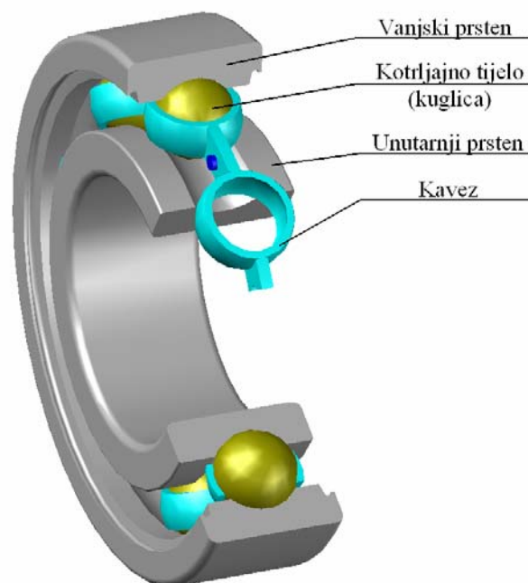
Slika 4.1 Radijalni kotrljajni kuglični ležaj
