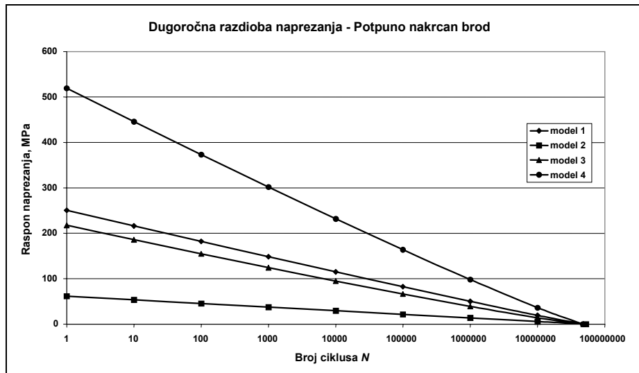
Slika 8-23 Dugoročna napreznja za detalje 1, 2, 3 i 4
