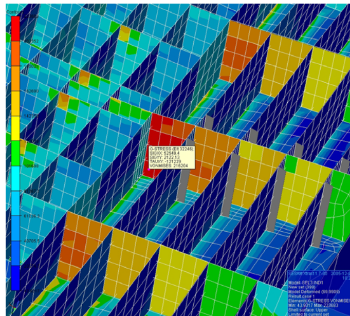
Slika 12-15 Ukupna naprezanja u dvodnu – Superelement 3 – Element 32246
