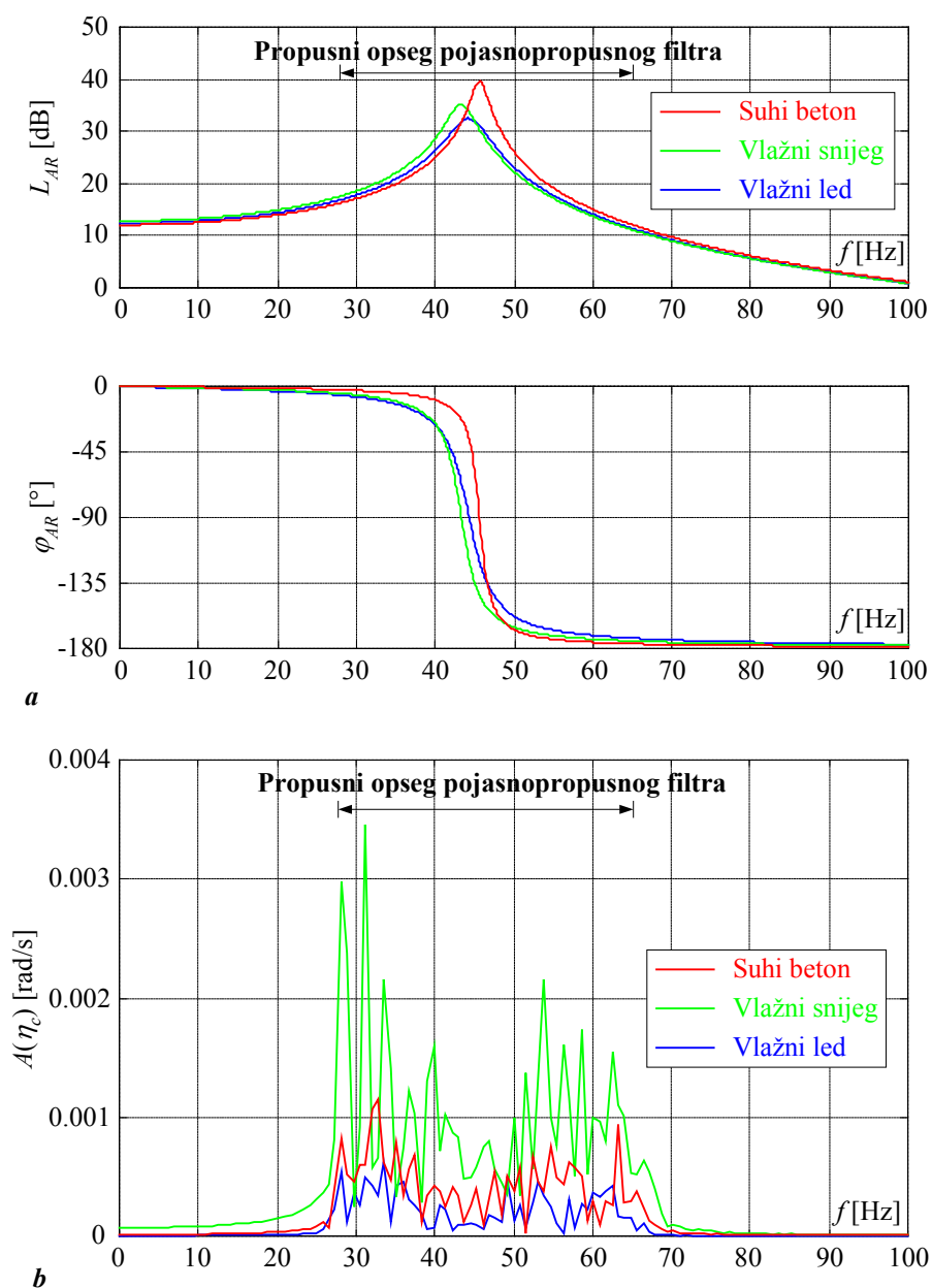
Slika 4.25. Frekvencijske karakteristike identificiranih AR modela torzijskih vibracija (a) i amplitudni spektri procijenjenog "obojenog" šuma (b) za vožnju po suhom betonu, vlažnom snijegu i vlažnom ledu ( v \approx 40 km/h, Ford Focus, ABS senzor).
