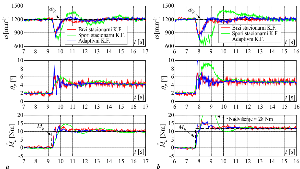
Slika 7.14. Usporedni eksperimentalni rezultati različitih ISC sustava s obzirom na skokovitu promjenu momenta tereta (udarno opterećenje) iznosa 10 Nm (a), i 12 Nm (b).
