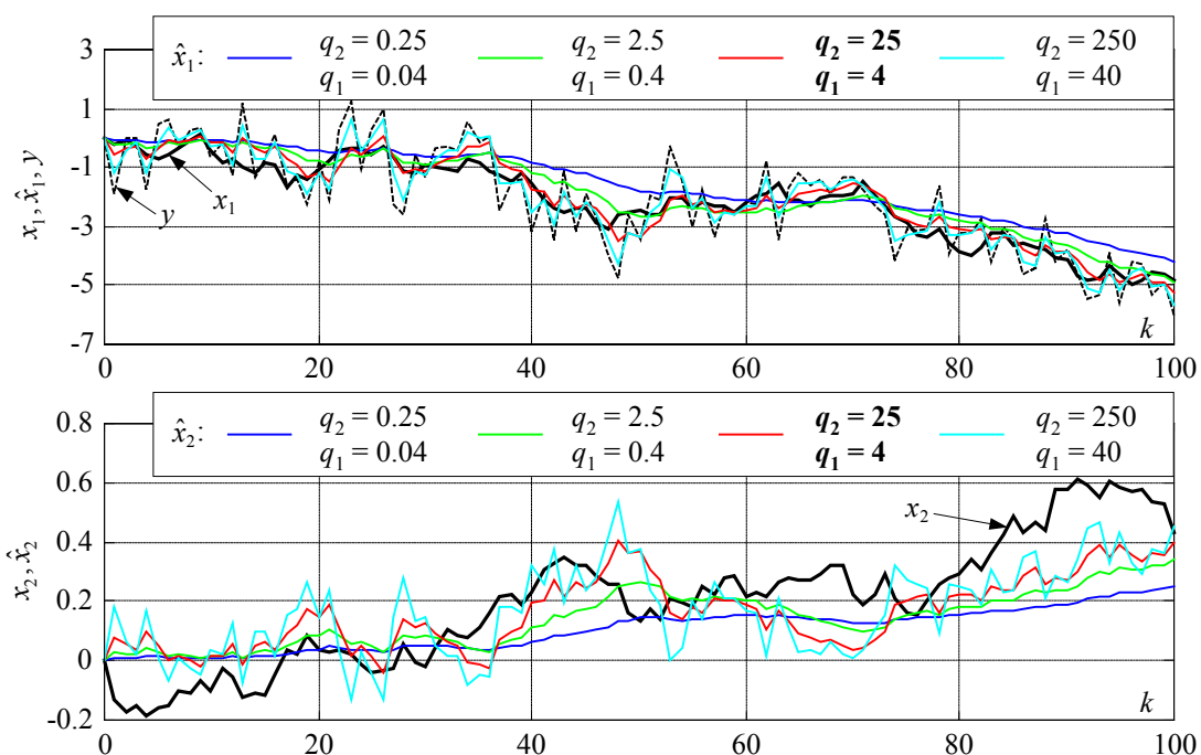
Slika 5.5. Usporedni odzivi Kalmanovog filtra za različite izbore matrice Q ( R = 1 ).
