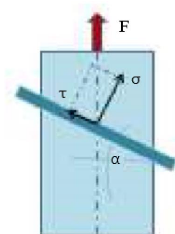
Slika 3-4. Jednoosno naprezanje [53].
