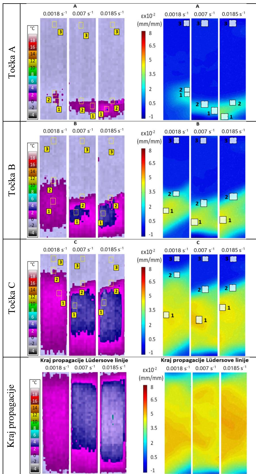
Slika 7-61. Kvalitativna analiza termografijom i digitalnom korelacijom slike pri brzinama deformacija v_1 , v_2 i v_3 u pozicijama 1, 2 i 3 točaka A-C i kraja propagacije Lüdersove linije.
