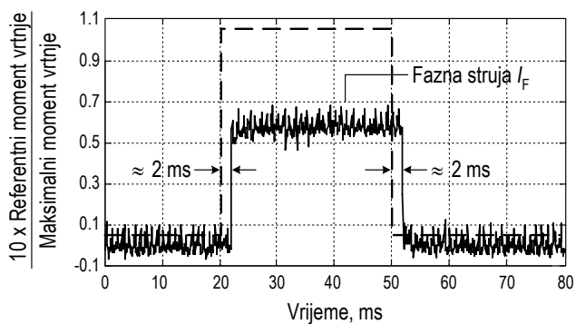
Slika 7.3 Odziv fazne struje motora za skokovitu promjenu momenta vrtanje uz zakočeni rotor motora ( n=0 ).
