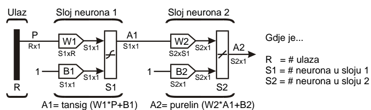
Slika 3.10. Shema dvoslojne unaprijedne backpropagation mreže [58]
