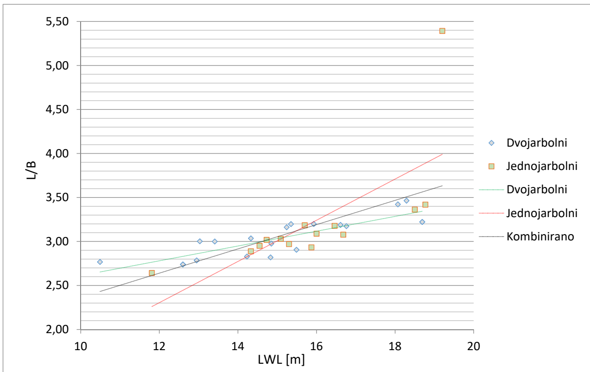
Slika 56. L/B - LWL
