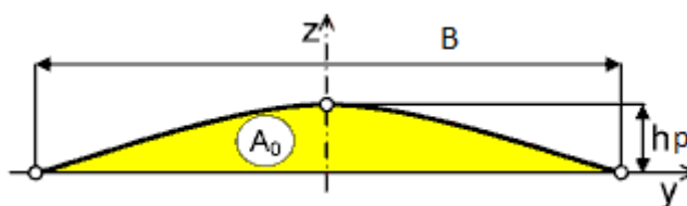
Slika 18. Preluk palube [15]
