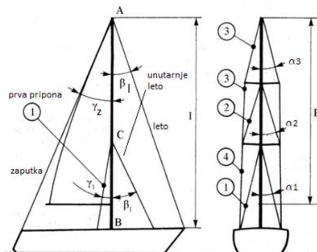
Slika 63. Kutevi opute [21]
