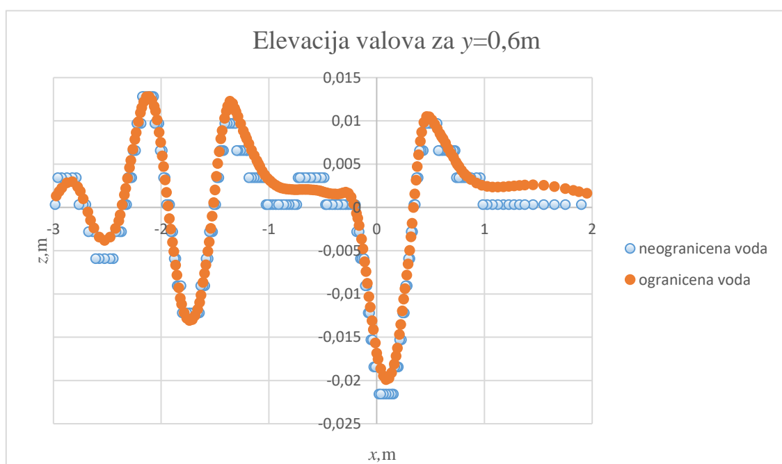
Slika 47. Elevacije valova u ravni y=0,6m za katamaran K3 za neograničenu i ograničenu vodu
