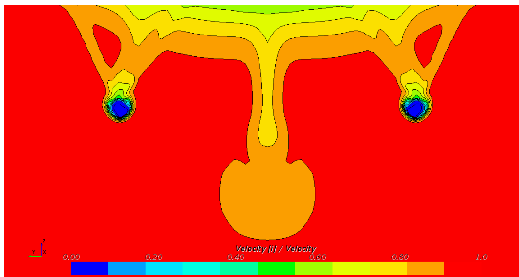
Slika 61. Polje nominalnog sustrujanja u ravni brodskog vijka (Model 2, RSM)
