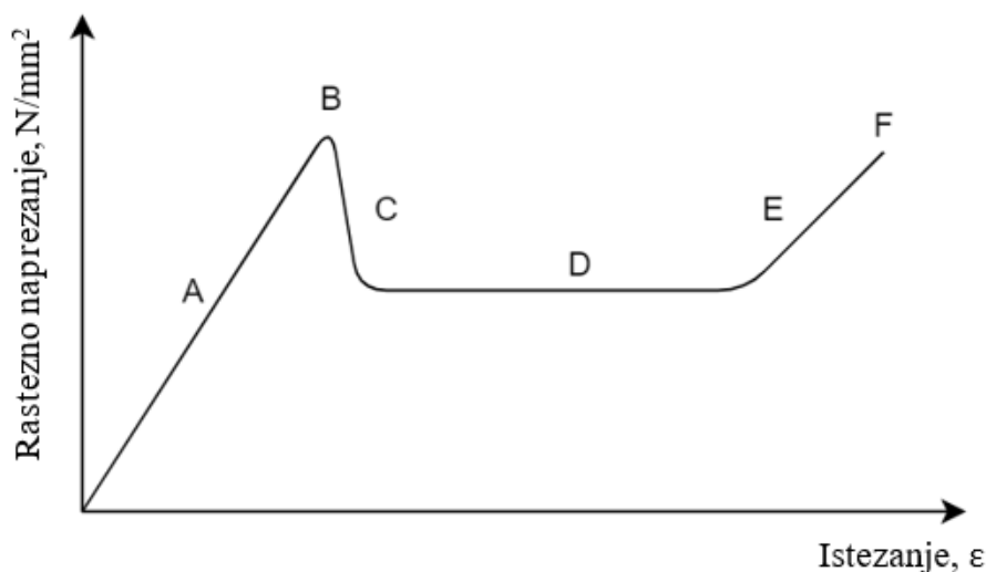
Slika 6.1. Opći oblik krivulje rasteznog napreznja-istežanja za polimerne materijale [47]
