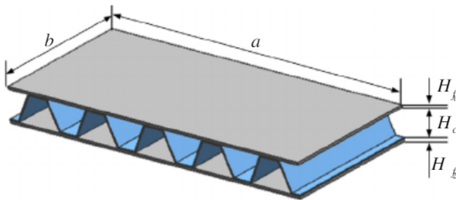
Slika 2.6: Trapezni sendvič panel [6]
