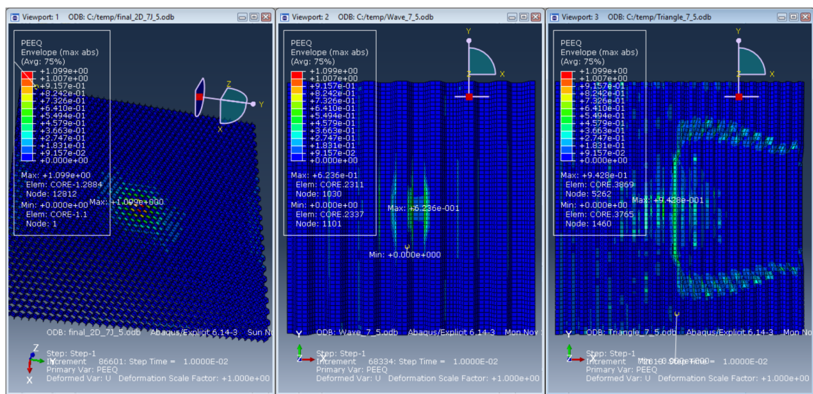
Slika 5.22: Raspodjela ekvivalentne plastične deformacije za energiju udara od 7 J i visinu jezgre od 5 mm
