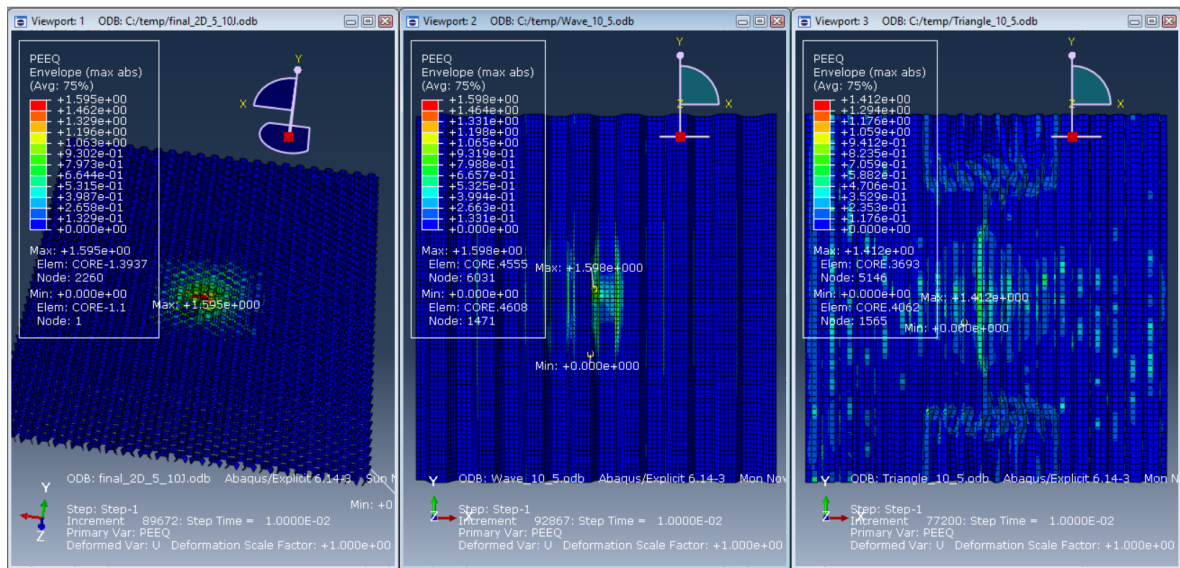
Slika 5.26: Raspodjela ekvivalentne plastične deformacije za energiju udara od 10 J i visinu jezgre od 5 mm
