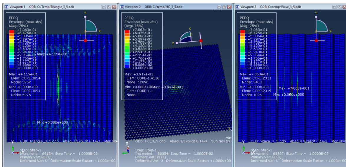
Slika 5.16: Raspodjela ekvivalentne plastične deformacije za energiju udara od 3 J i visinu jezgre od 5 mm
