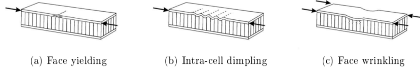
Slika 2.1: Načini popuštanja vanjskih slojeva,
