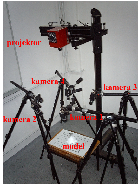
Slika 8.1. Postava sustava
