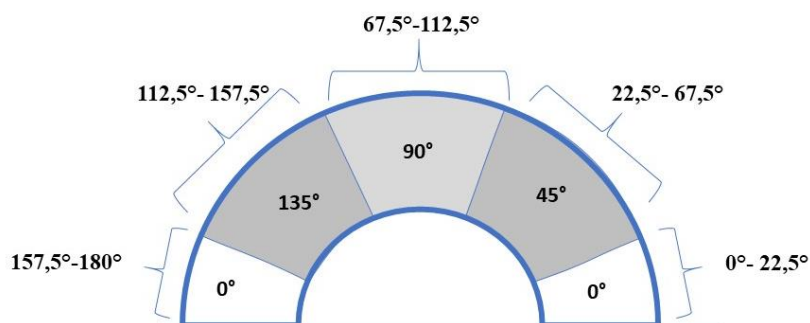
Slika 4.5 Određivanje orijentacije ruba Cannyevim postupkom [21]
