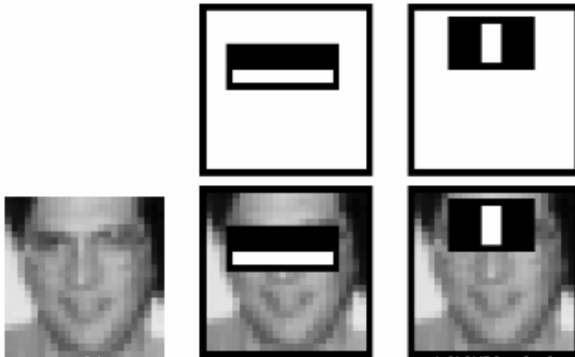
Slika 44. Integralne slike
