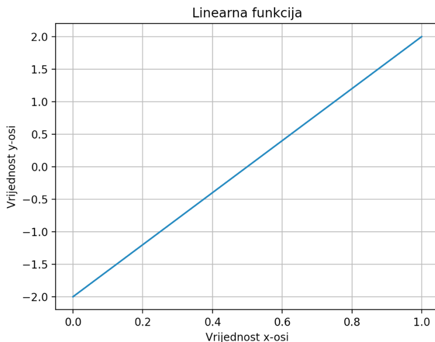
Slika 21. Linearna funkcija
