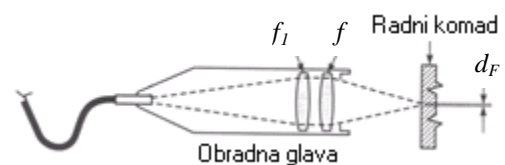
d) fokusiranje snopa.
