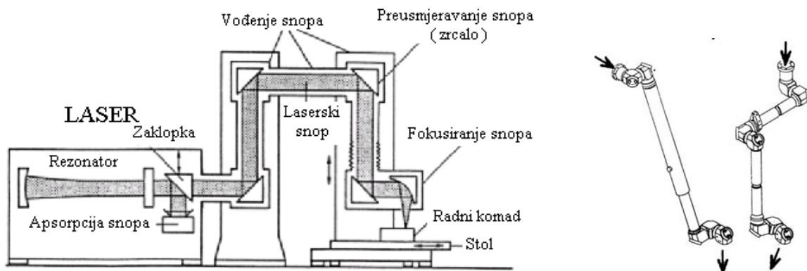
a) fiksna zrcala.
