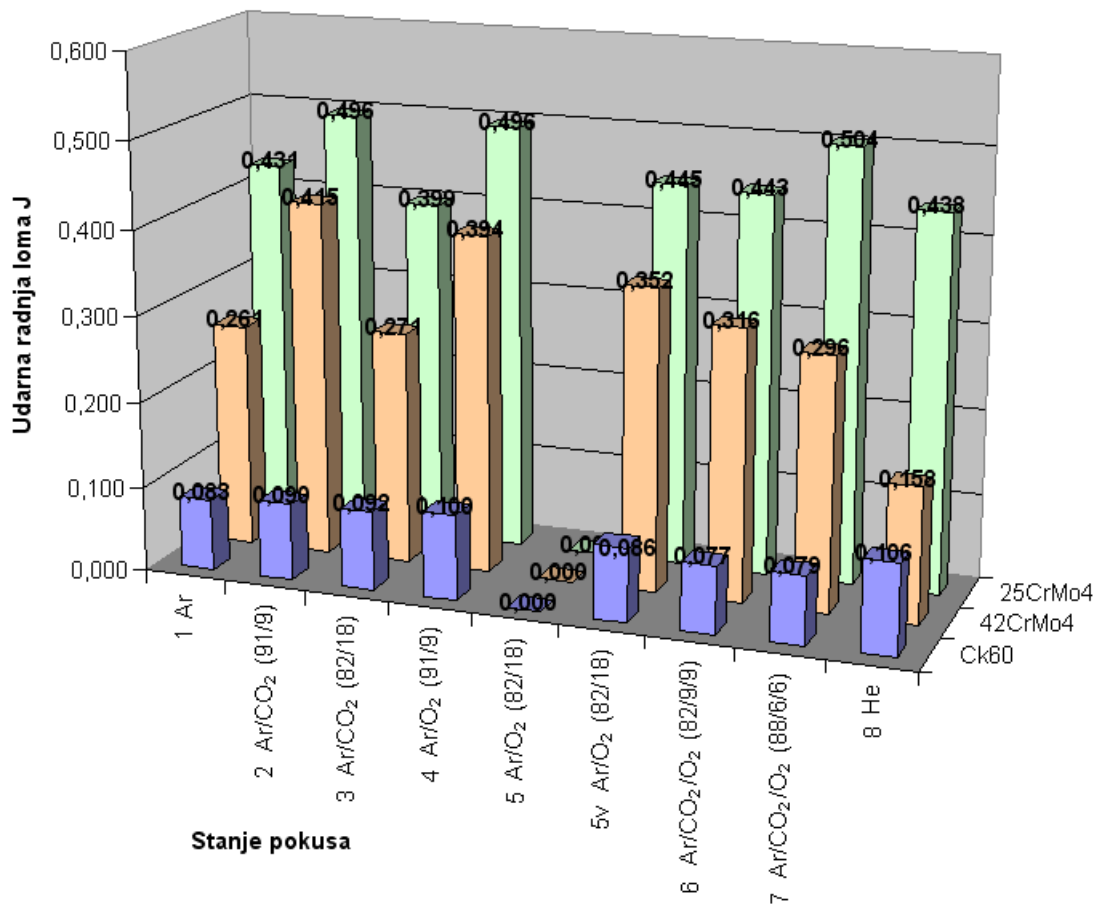
Slika 63. Udarne radnje loma dobivene Zgaginom metodom.
