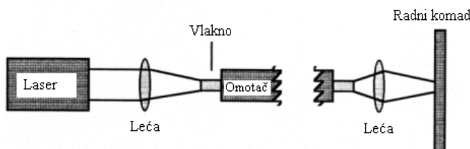
c) princip vođenja snopa kroz optičko vlakno.
