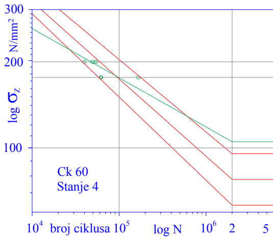
c) Stanje pokusa 4 - Ar/O 2 (91/9).
