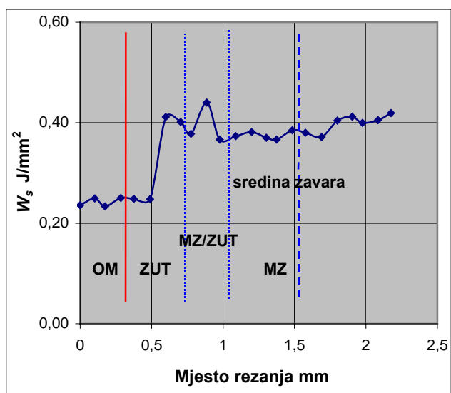
Slika 69. Profili mehaničkih svojstava zavarenog spoja – 2 Ar/CO 2 (91/9).
