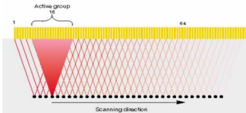
Slika 21: Shematski prikaz elektroničkog skeniranja [5]
