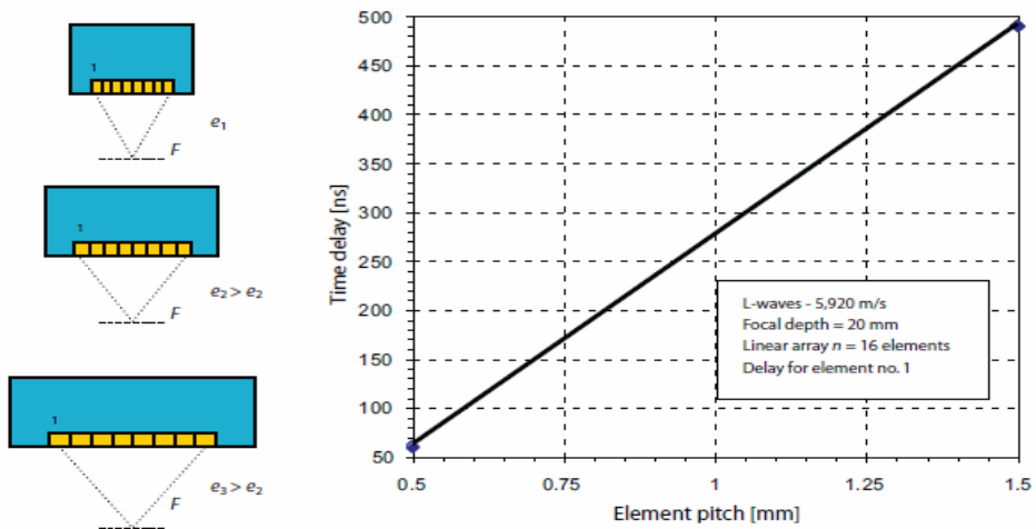
Slika 7: Ovisnost zadržke o veličini pretvornika kod iste žarišne udaljenosti [1]
