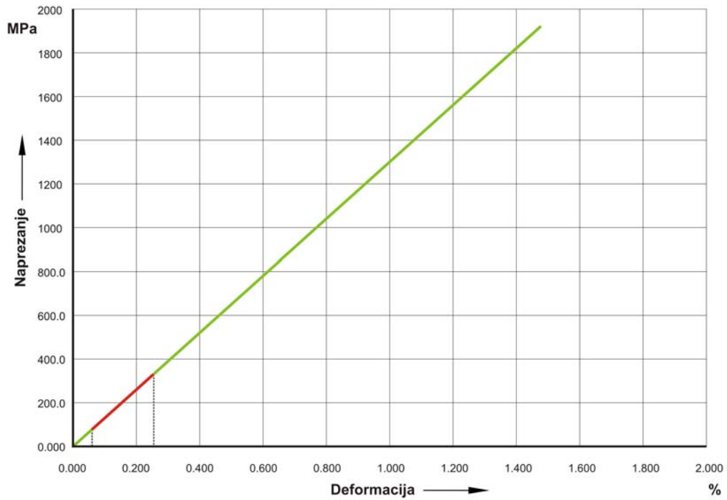
Slika 2.7 Dijagram \sigma - \varepsilon CFRP kompozita opterećenog u smjeru vlakana (eproveta 1)
