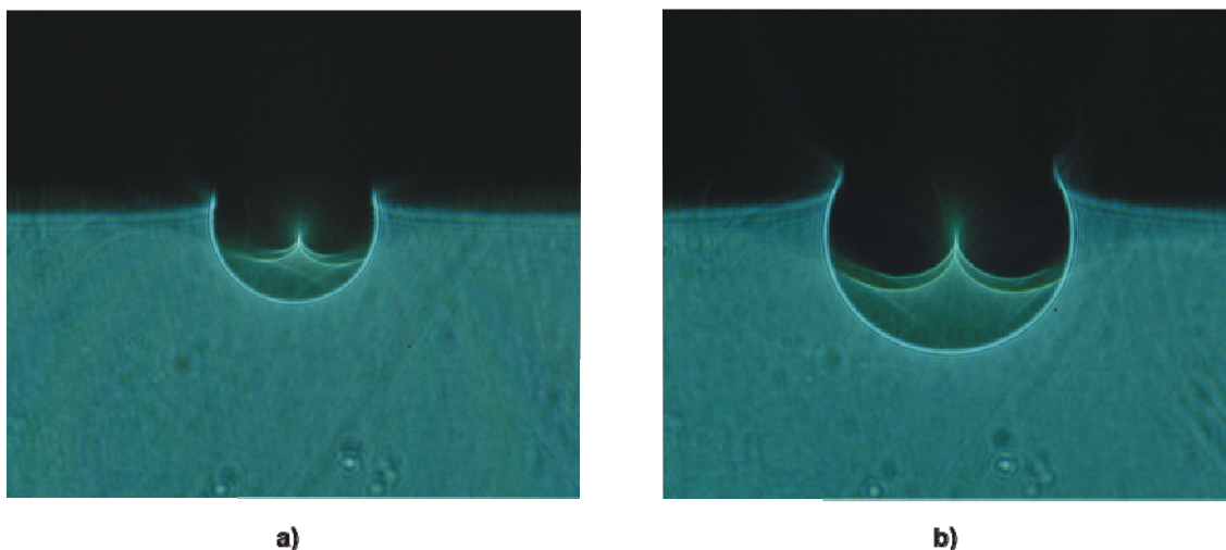
Slika 5.11 Utjecaj iznosa sile opterećenja na oblik i veličinu kaustike.
