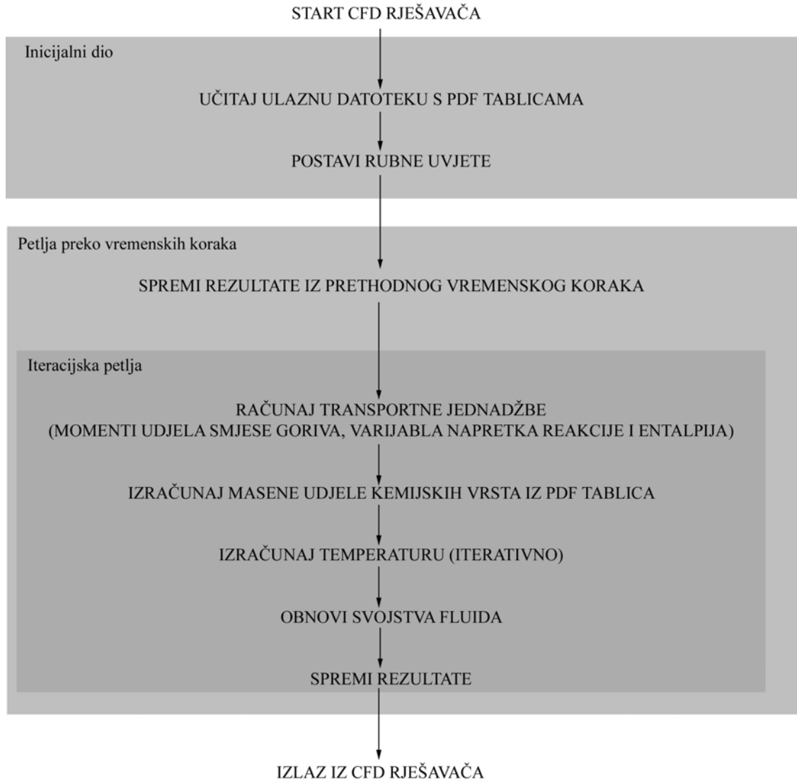
Slika 25 – Implementacija modela izgaranja (shema)
