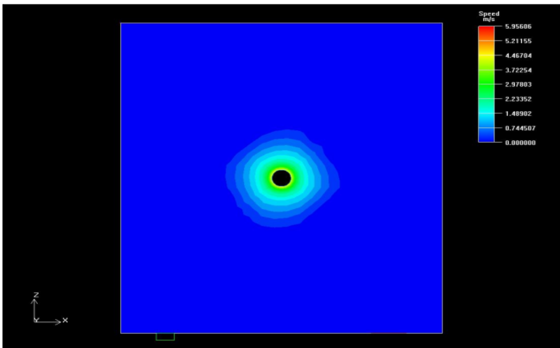
Slika 17. Prikaz kontura brzina na istrujnoj površini vrtložnog stropnog difuzora
