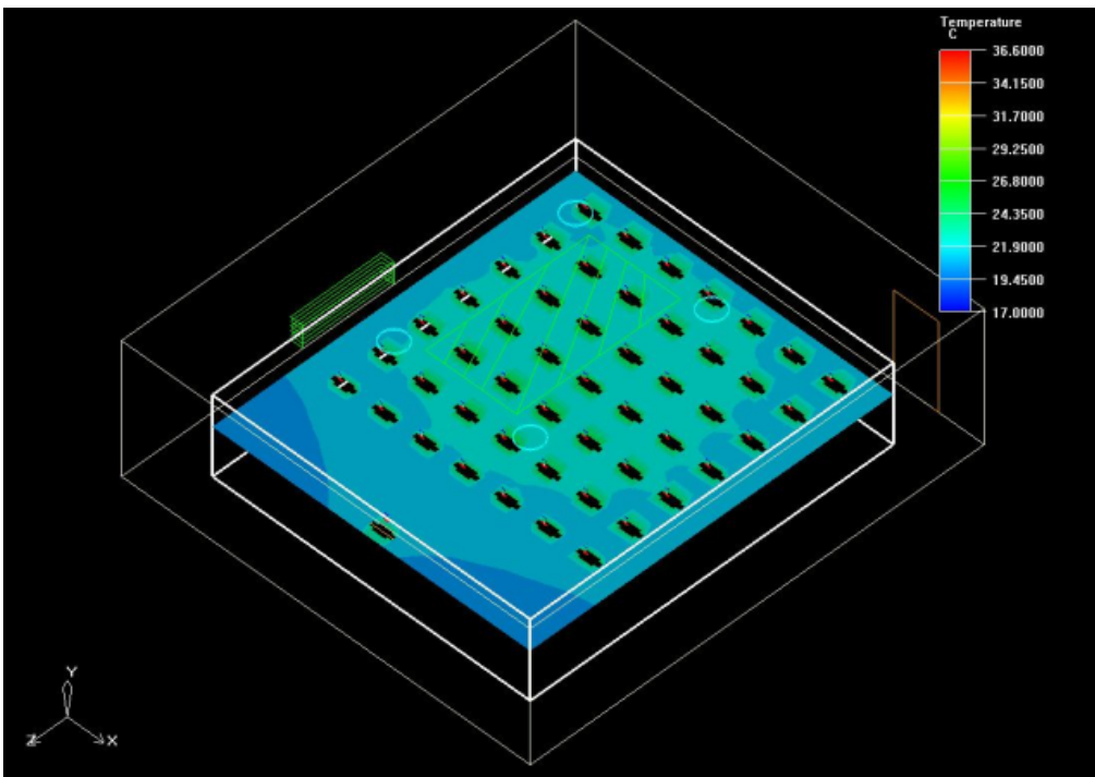
Slika 29. Izometrijski prikaz distribucije temperature zraka u ravni udaljenoj 110 cm od poda
