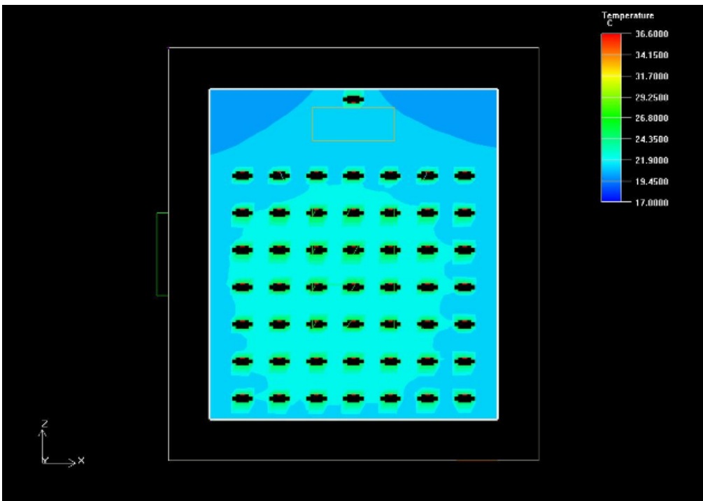
Slika 30. Tlocrtni prikaz distribucije temperature zraka u ravni udaljenoj 110 cm od poda
