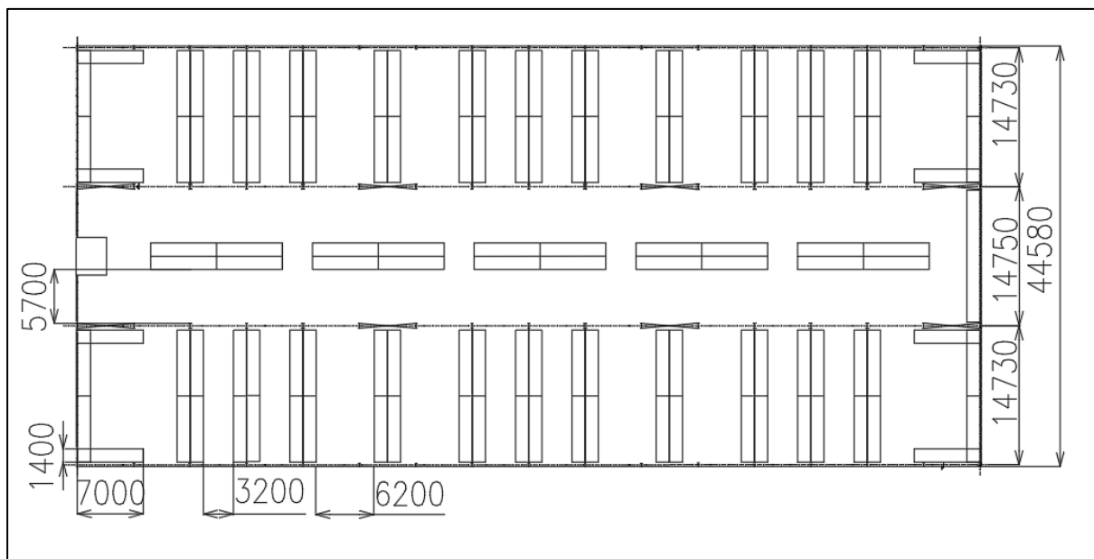
Slika 7.7 Paletni regali jednostruke dubine, okomiti na glavni prolaz
