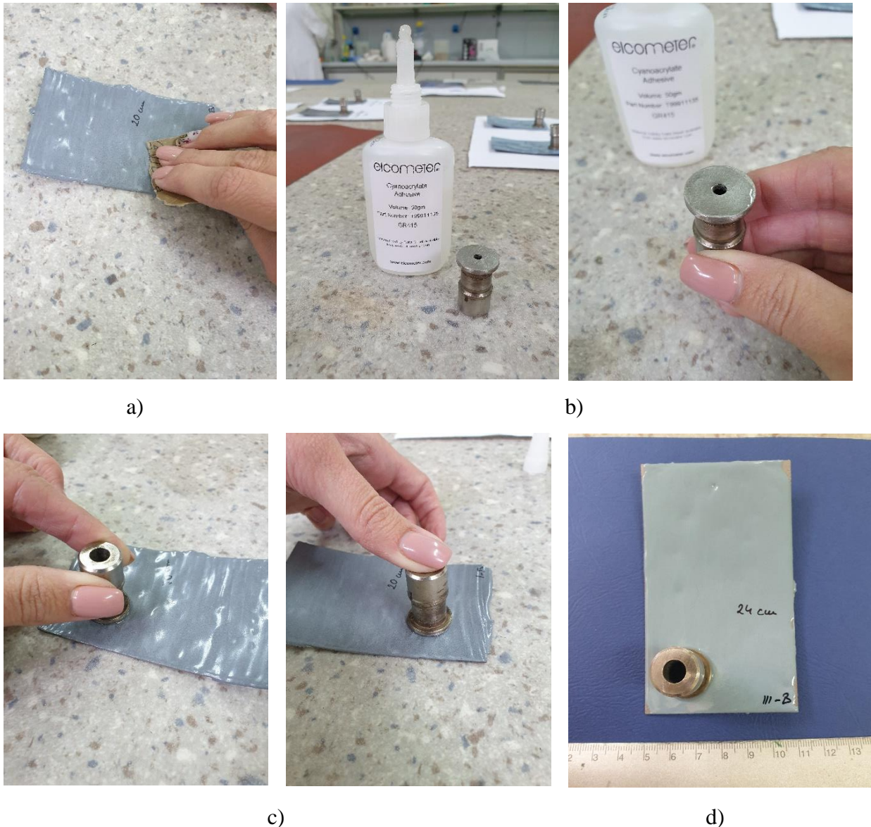
Slika 7.36. Postupak pripreme za Pull – off ispitivanje: a) hrapavljenje površine brusnim papirom, b) korišteno ljepilo te njegovo nanošenje, c) prislanjanje valjčića na površinu premaza, d) stvrdnjavanje ljepila
