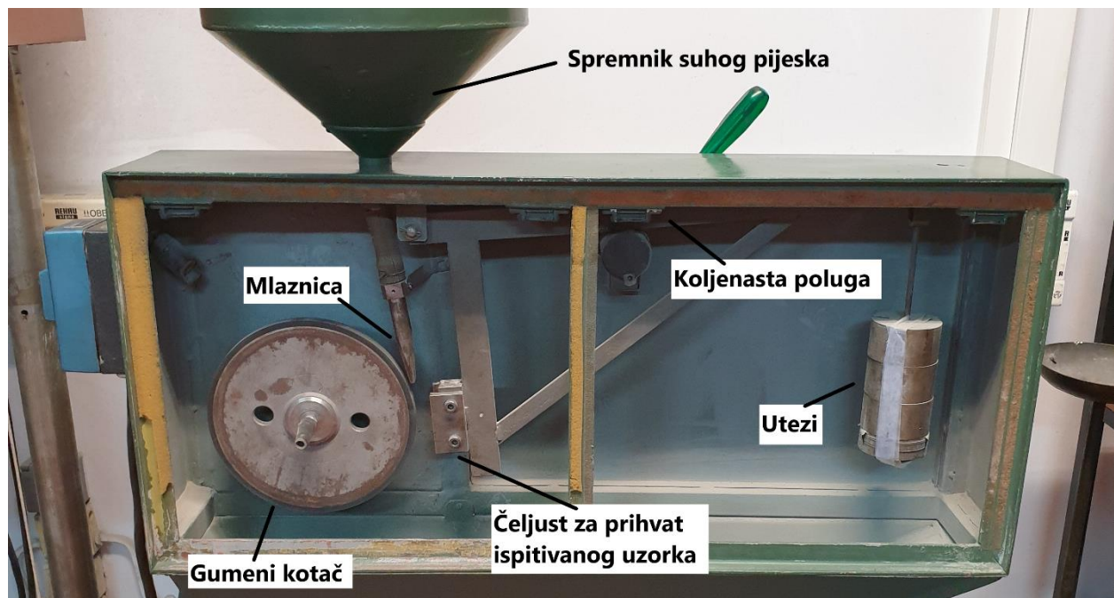
Slika 7.25. Dijelovi uređaja za ispitivanje otpornosti na abrazivsko trošenje
