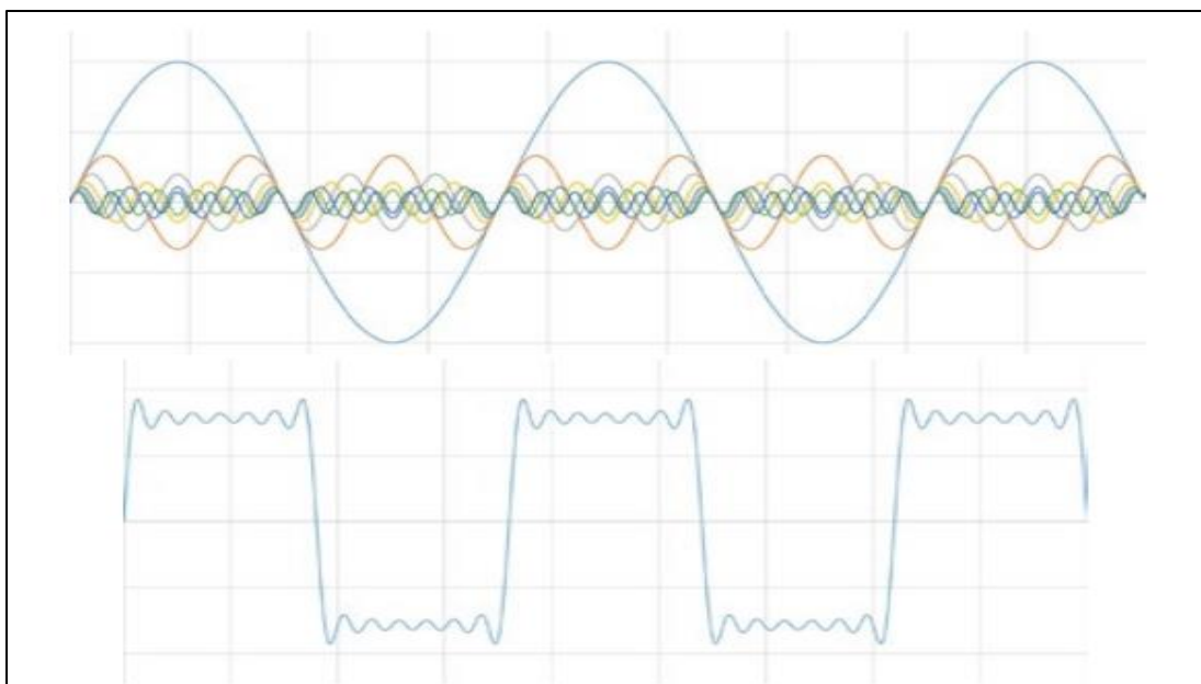
Slika 10. Pravokutni val kao suma sinusoida [7]
