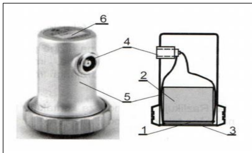
Slika 4. Dijelovi ravne sonde [2]
