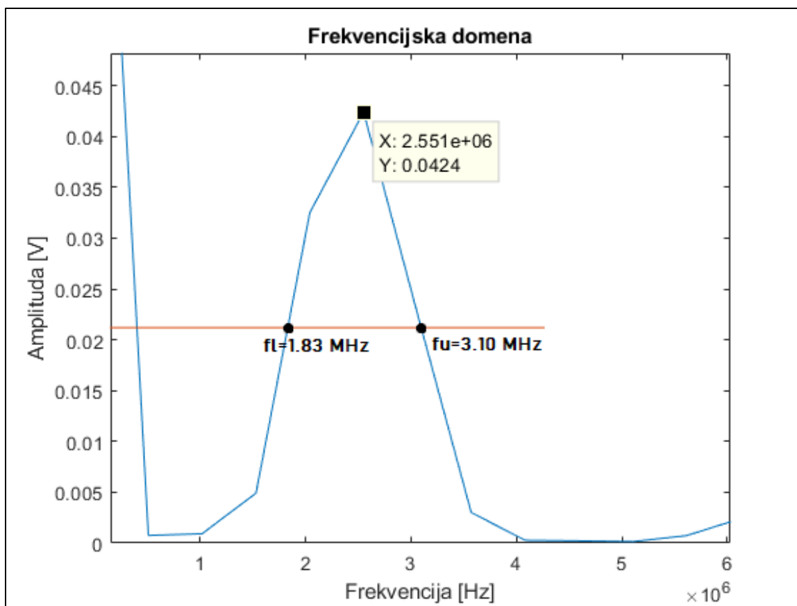
Slika 34. Frekvencijska domena signala snimljenog na etalonu V1 sondom MB2S
