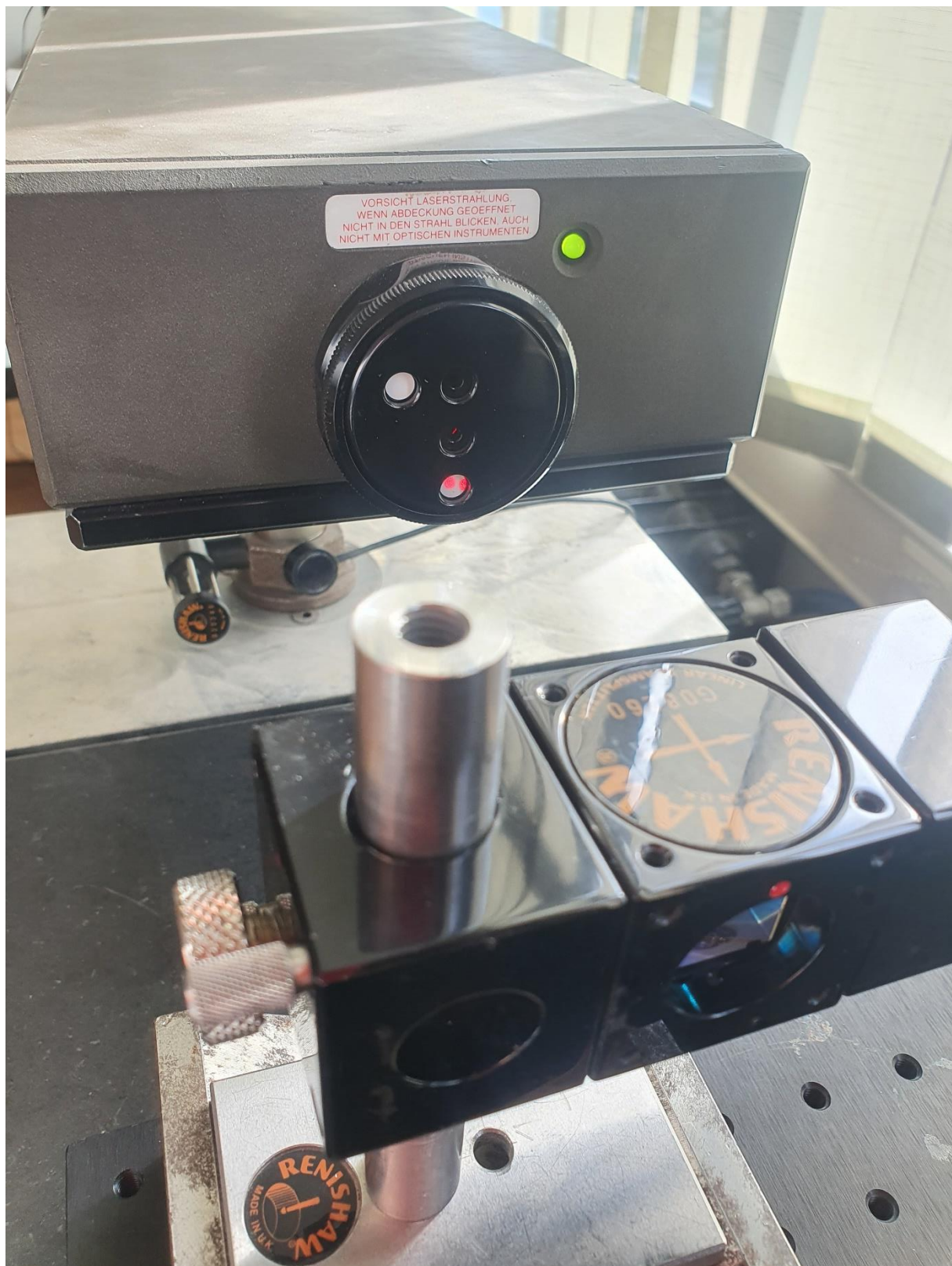
Slika 33 Neporavnati razdjelnik snopova sa retroreflektorom
