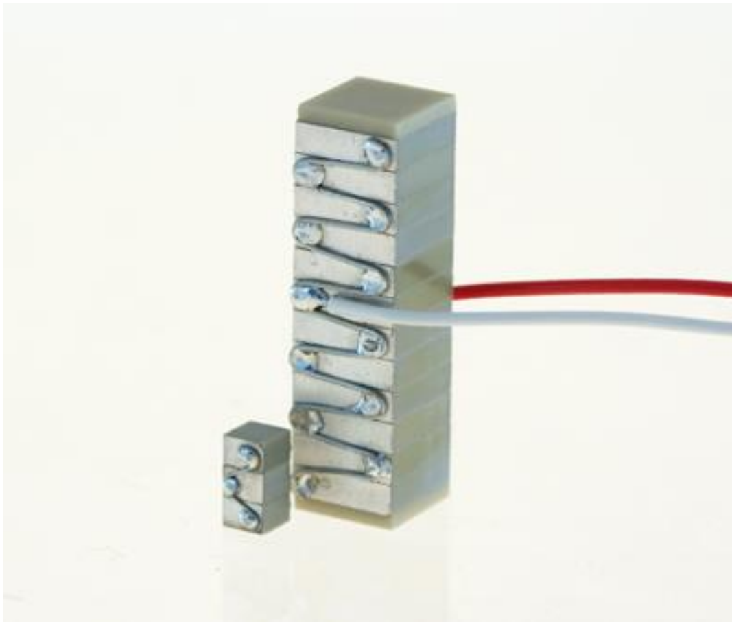
Slika 5 Uzdužni aktuator
