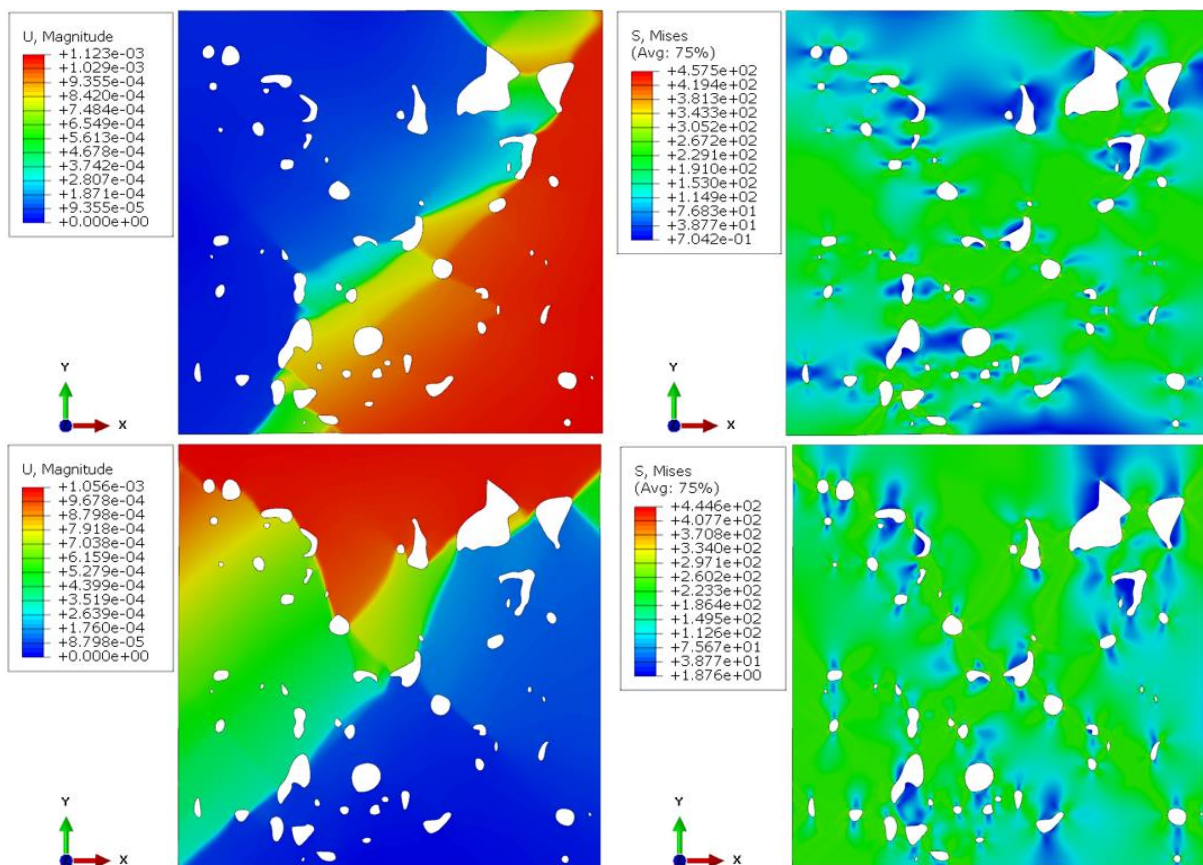
Slika 5.8 – Polje pomaka [mm] (lijevo) i ekvivalentnog von Misesovog naprezanja [MPa] (desno) za horizontalni (gore) i vertikalni (dolje) vlačni test i RVE dimenzija 0,2x0,2 mm
