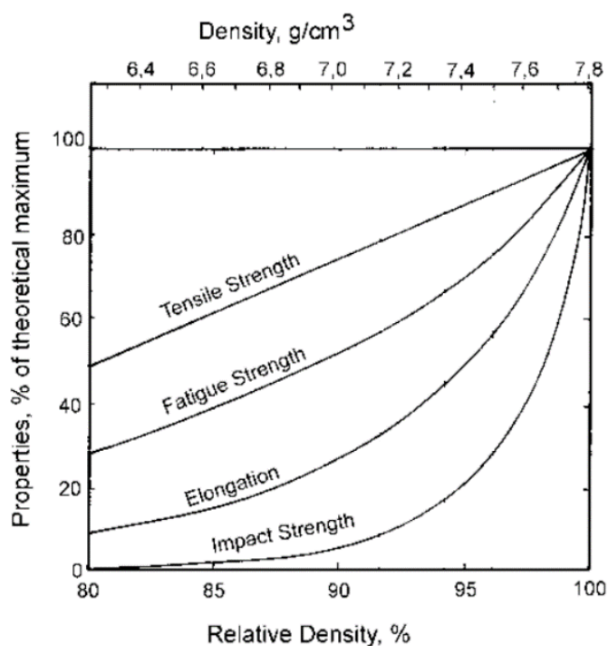
Slika 1.3 – Utjecaj gustoće na mehanička svojstva [6]
