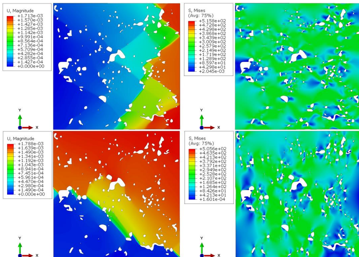
Slika 5.9 – Polje pomaka [mm] (lijevo) i ekvivalentnog von Misesovog naprezanja [MPa] (desno) za horizontalni (gore) i vertikalni (dolje) vlačni test i RVE dimenzija 0,3x0,3 mm
