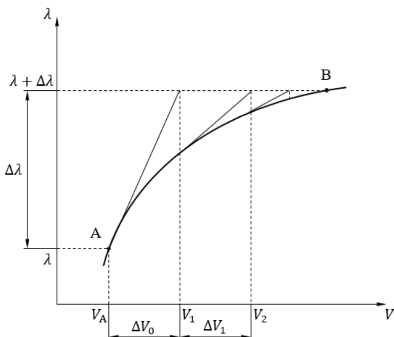
Slika 3.3 – Newton-Raphsonova metoda
