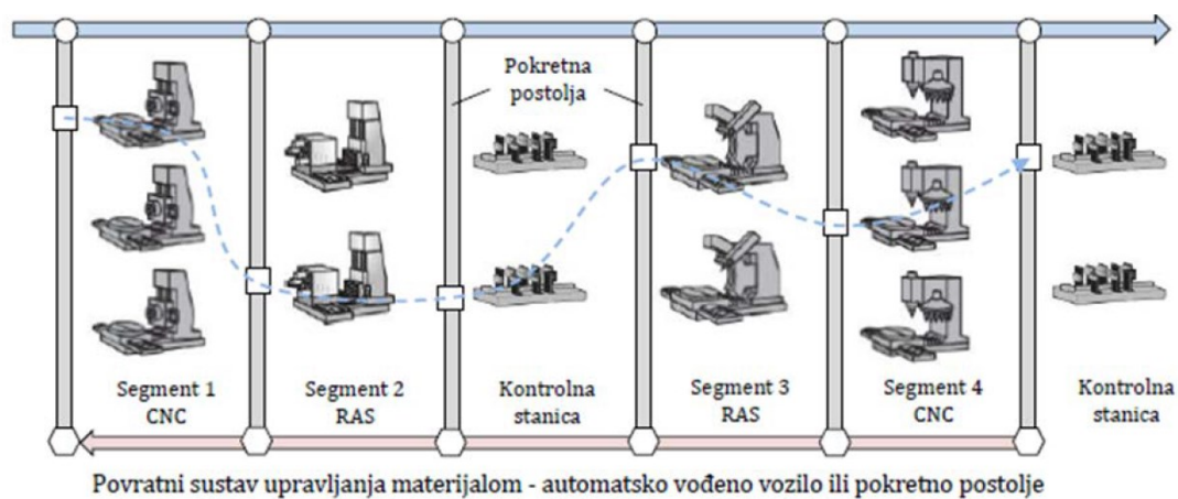
Slika 14. Shema rekonfigurabilnog proizvodnog sustava [13]
