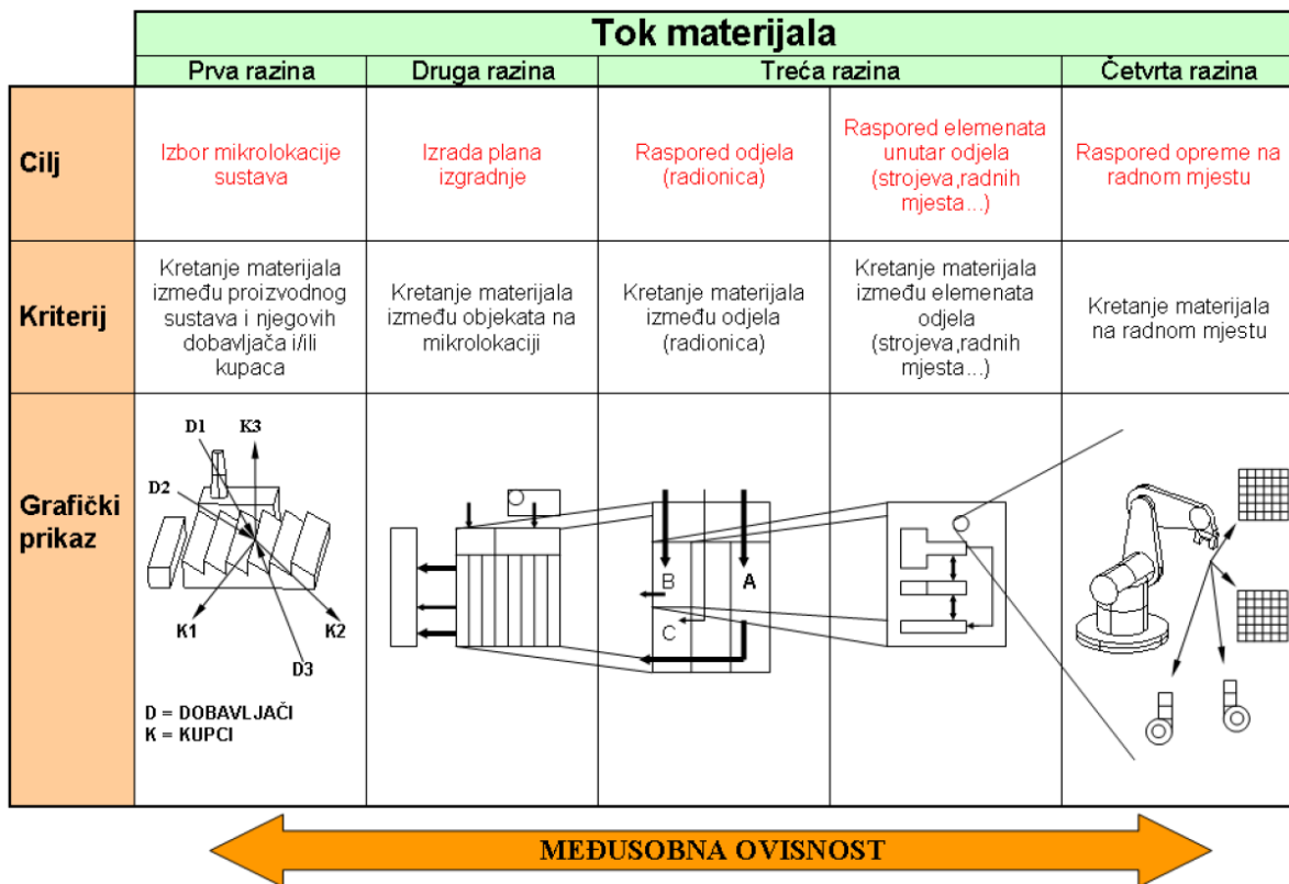
Slika 5. Razine toka materijala [3]
