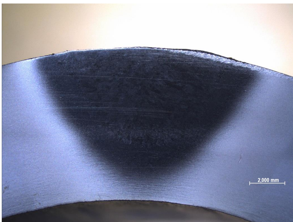
Slika 49. Makroizbrusak uzorka 2
