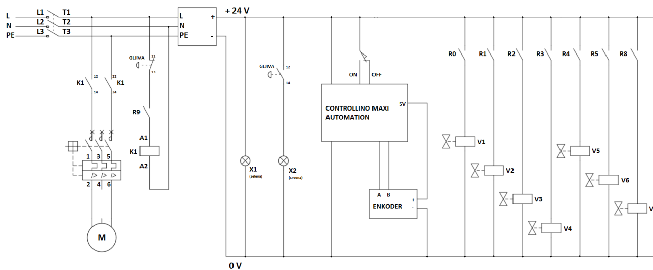
Slika 44. Električna shema
