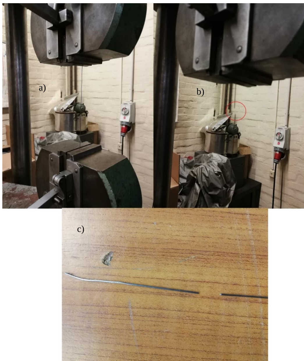
Slika 3.17 Statičko vlačno ispitivanje čelične žice
