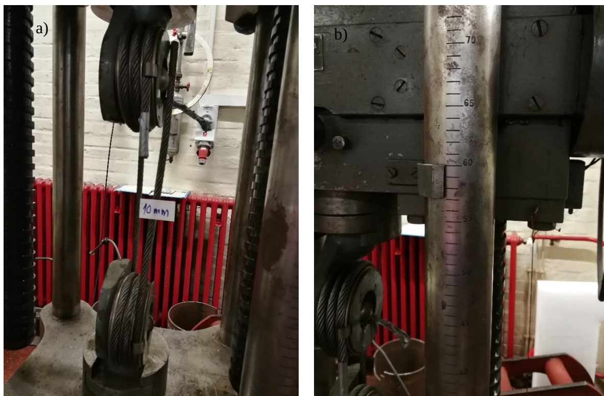
Slika 3.6 Užde u početnoj poziciji ispitivanja i očitavanje pomaka čeljusti
