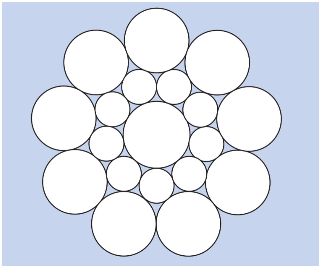
Slika 2.10. Konstrukcija kabela Seale [5]
