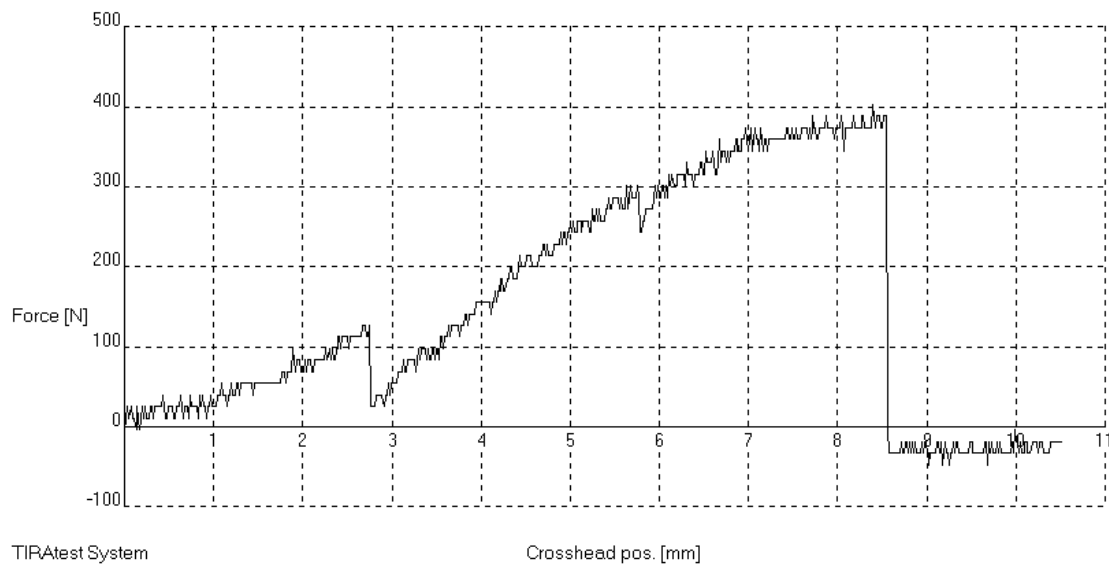
Slika 3.18 Dijagram sila-pomak jednog uzorka žice iz užadi promjera 8 mm (proizvođač A)
