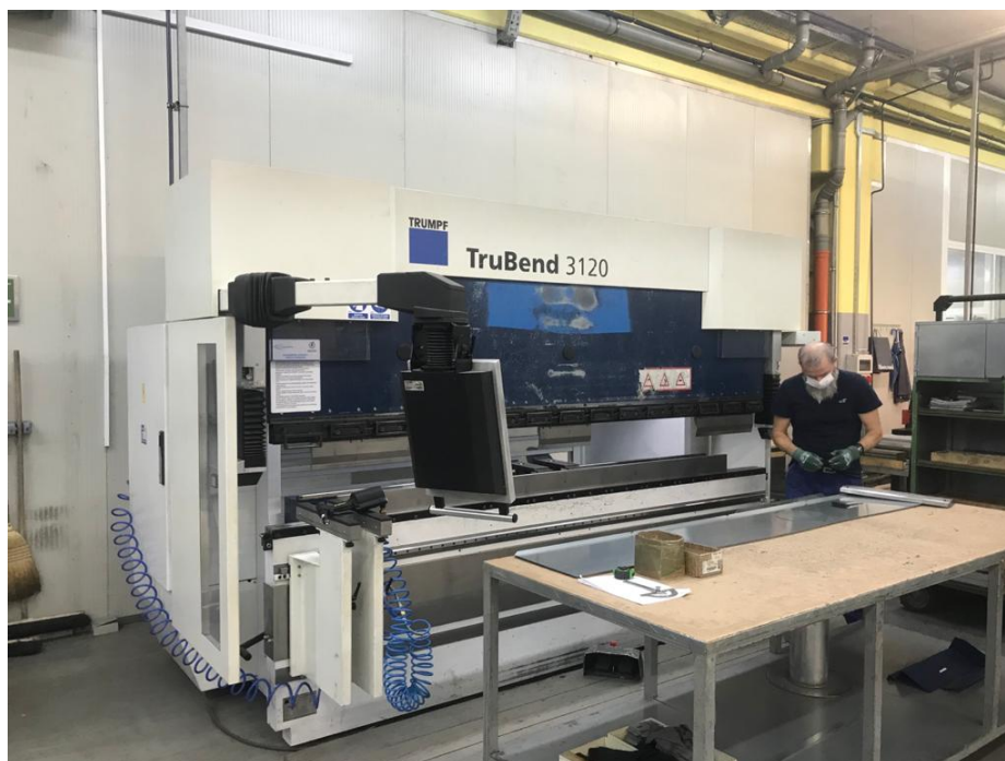
Slika 38. TruBend 3120 CNC savijačica
