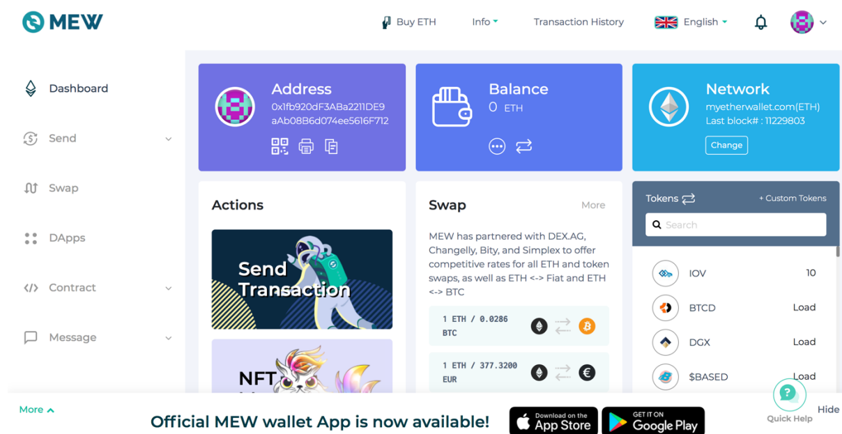
Slika 43. Ethereum novčanik
