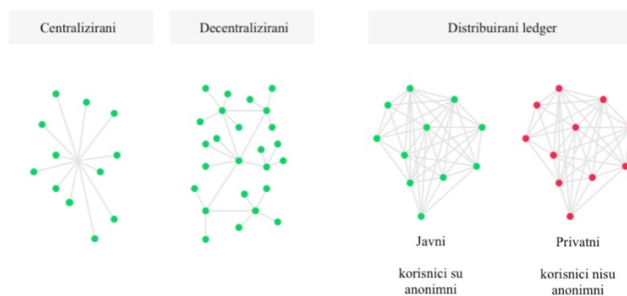
Slika 18. Arhitektura blockchaina [13]
