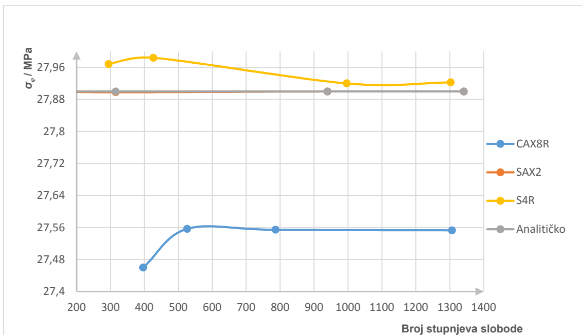
Slika 50. Konvergencija cirkularnog naprežanja za različite elemente
