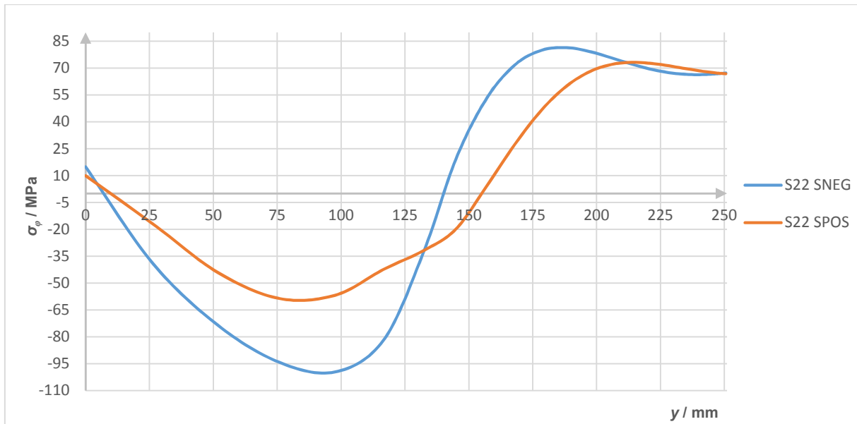
Slika 80. Raspodjela cirkularnih naprezanja duž vanjskog i unutarnjeg ruba torisferne ljsuske - tlačna proba
