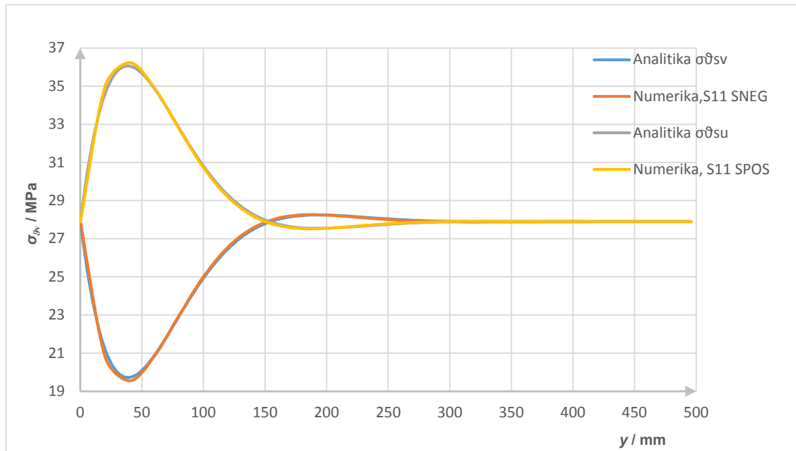
Slika 59. Raspodjela meridijalnih naprezanja duž vanjskog i unutrašnjeg ruba sferne ljuske
