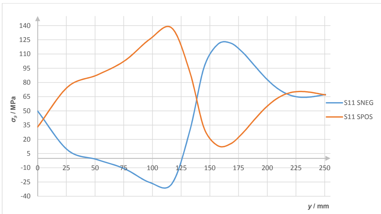
Slika 79. Raspodjela meridijalnih napreznja duž vanjskog i unutarnjeg ruba torisferne ljsuske - tlačna proba
