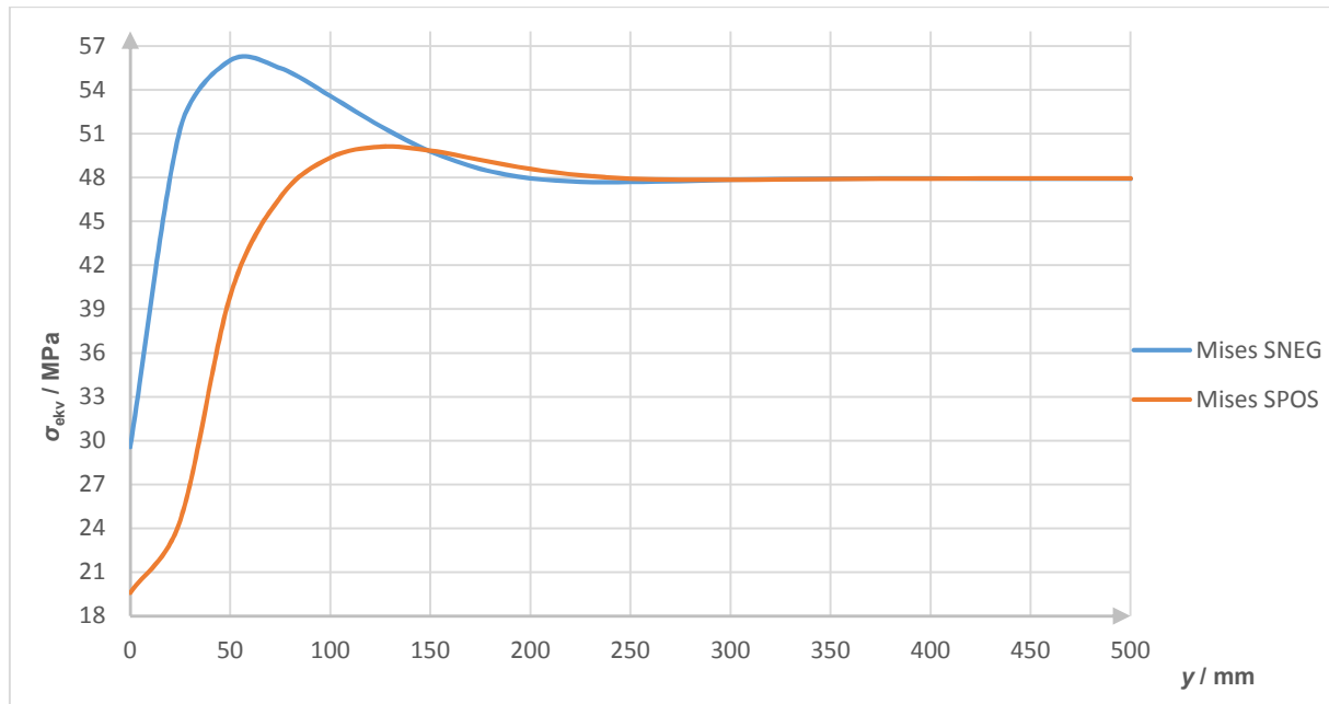
Slika 75. Raspodjela ekvivalentnog napreznja duž vanjskog i unutarnjeg ruba cilindrične ljuste - radno opterećenje
