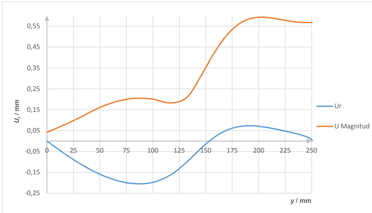
Slika 78. Raspodjela radijalnog pomaka torisferne ljsuske - tlačna proba
