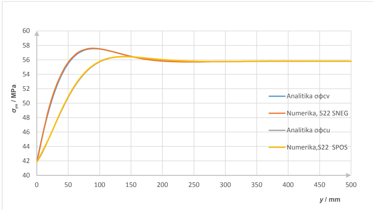
Slika 62. Raspodjela cirkularnog napreznja duž vanjskog i unutrašnjeg ruba cilindrične ljuske
