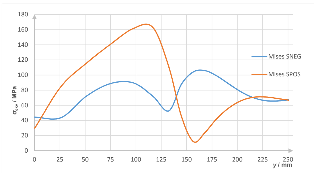
Slika 81. Raspodjela ekvivalentnog naprezanja duž vanjskog i unutarnjeg ruba torisferne ljsuske - tlačna proba
