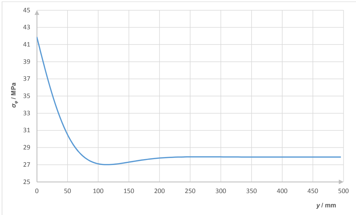
Slika 14. Raspodjela cirkularnog naprezanja sferne ljske
