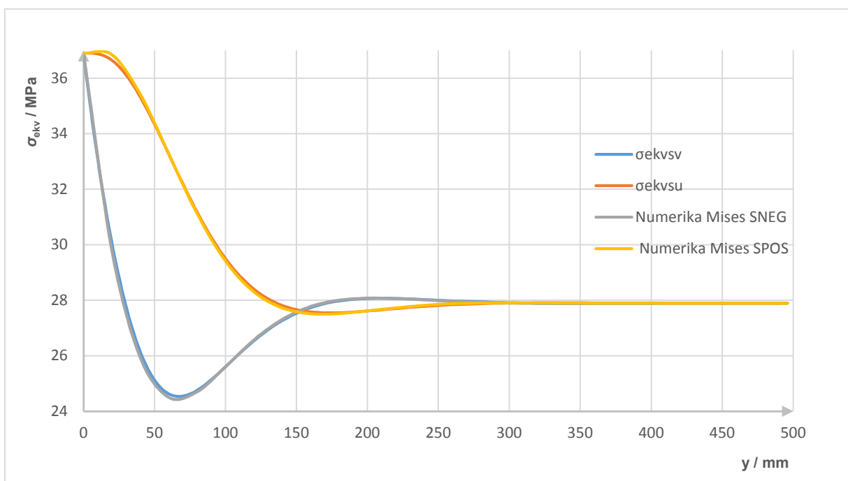
Slika 63. Raspodjela ekvivalentnog napreznja duž unutrašnjeg i vanjskog ruba sferne ljuske
