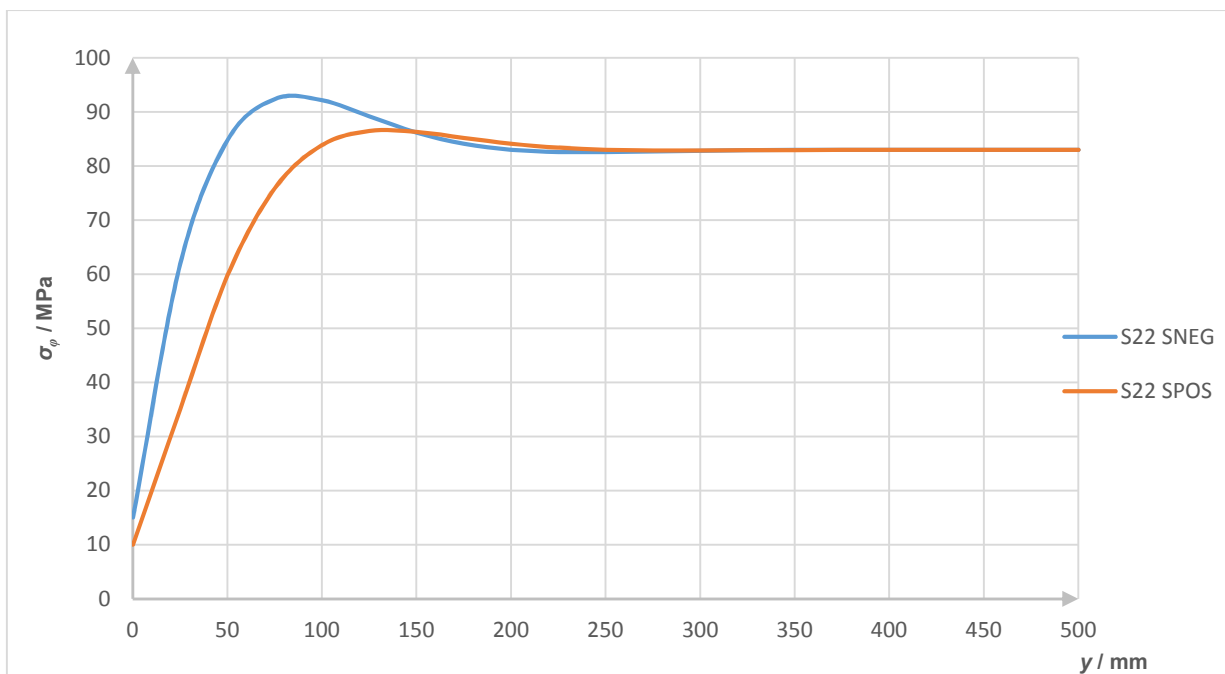
Slika 84. Raspodjela cirkularnih napreznja duž vanjskog i unutarnjeg ruba cilindrične ljsuke - tlačna proba
