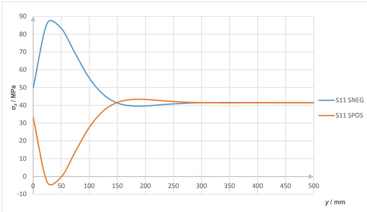
Slika 83. Raspodjela meridijalnih napreznja duž vanjskog i unutarnjeg ruba cilindrične ljsuke - tlačna proba
