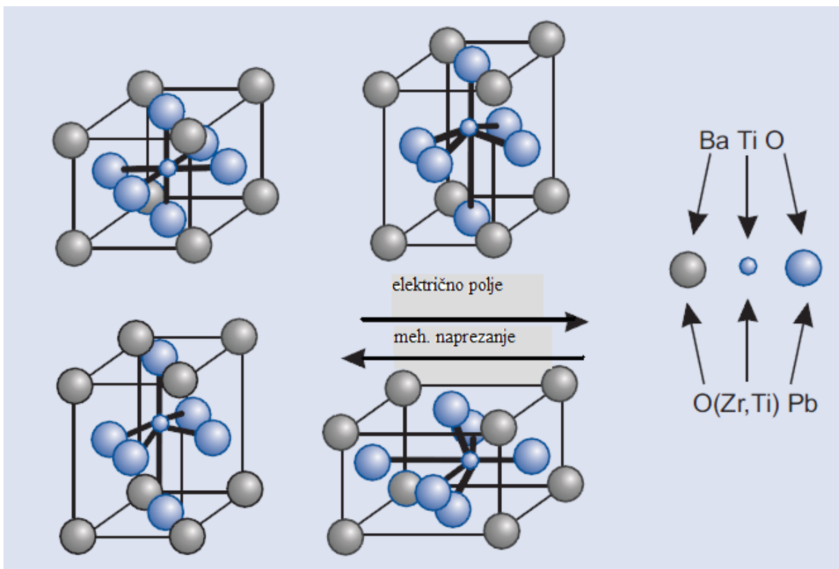
Slika 8. Struktura PZT i BaTiO 3 prije i nakon što je električno polje dovedeno na kristal, [10]
