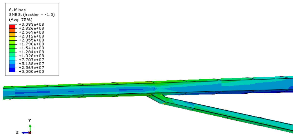
Slika 55. Von Misesova napreznja na zadnjoj ramenjači u blizini spoja, SBW [Pa]
