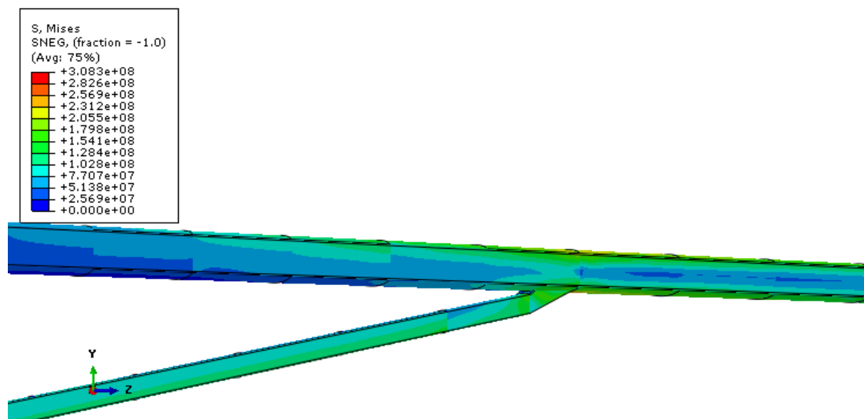
Slika 54. Von Misesova napreznja na prednjoj ramenjači u blizini spoja, SBW [Pa]
