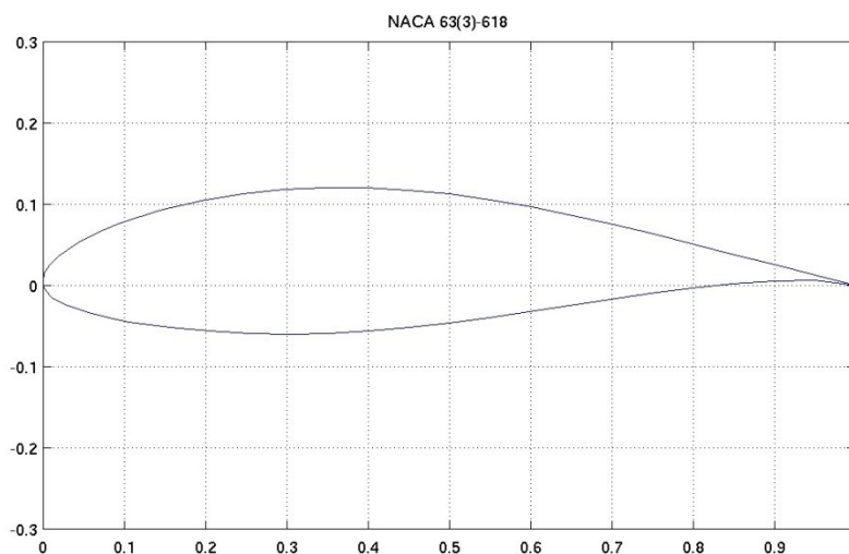
Slika 29. NACA 63(3)-618 [29]
