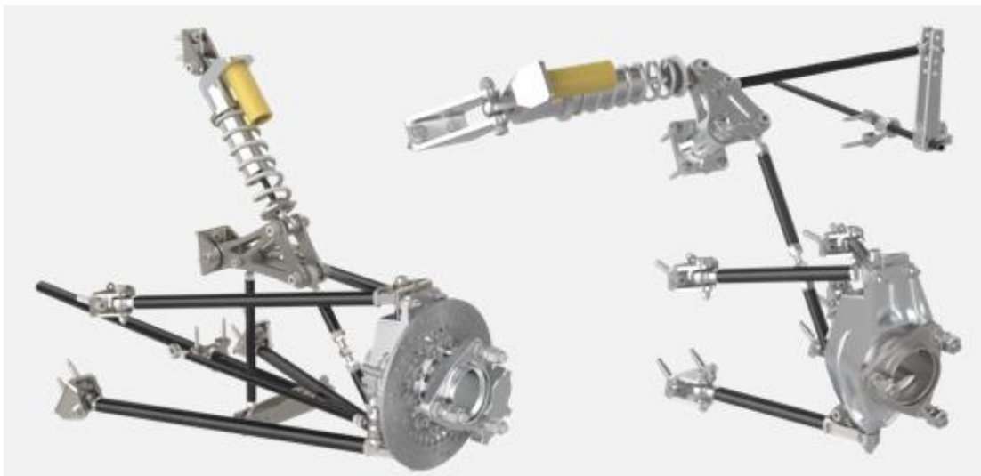
Slika 24: Prikaz ovjesa- prednji (lijevo) istražnji (desno)
