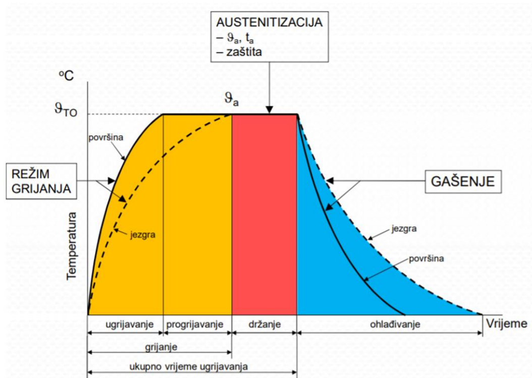
Slika 5: Postupak kaljenja [7]
