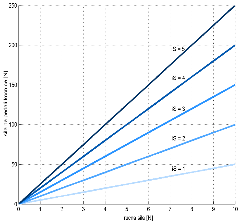
Slika 12. Odnos ručne sile i sile na pedali kočnice
