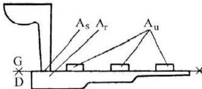
Slika 20. Semitlačni uljevni sustav [1]
