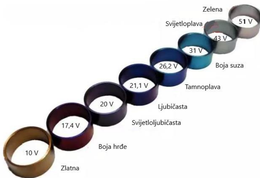
Slika 23. Ovisnost boje o naponu [25]
