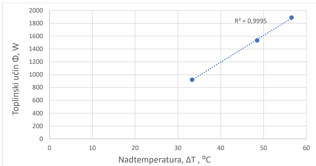
Slika 8. Karakteristična jednađba radijatora Global
