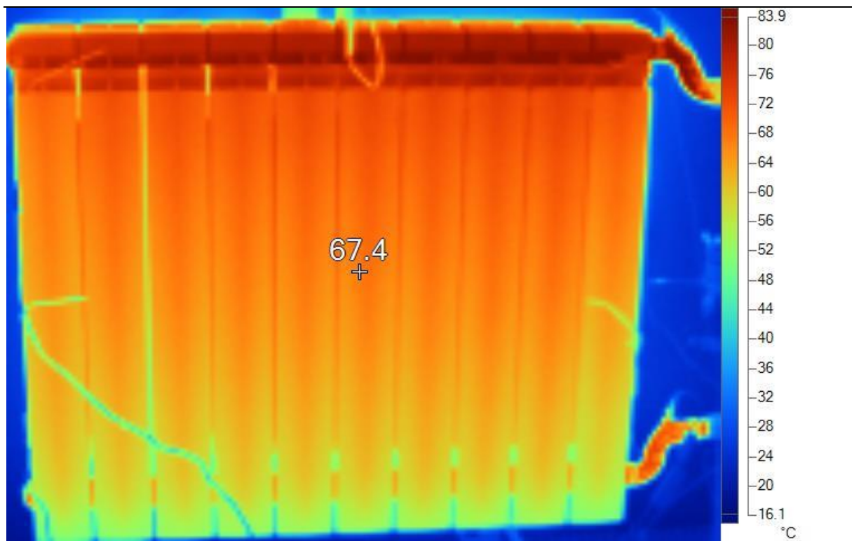
Slika 9. Termogram, radiator Lipovica, režim 85/75
