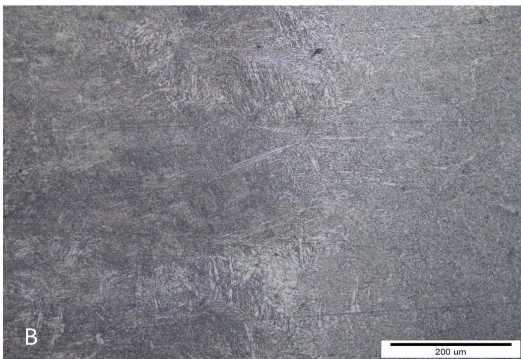
Slika 51. Mikroskopska snimka metala zavara i ZUT-a površine B pod uvećanjem 200 puta
